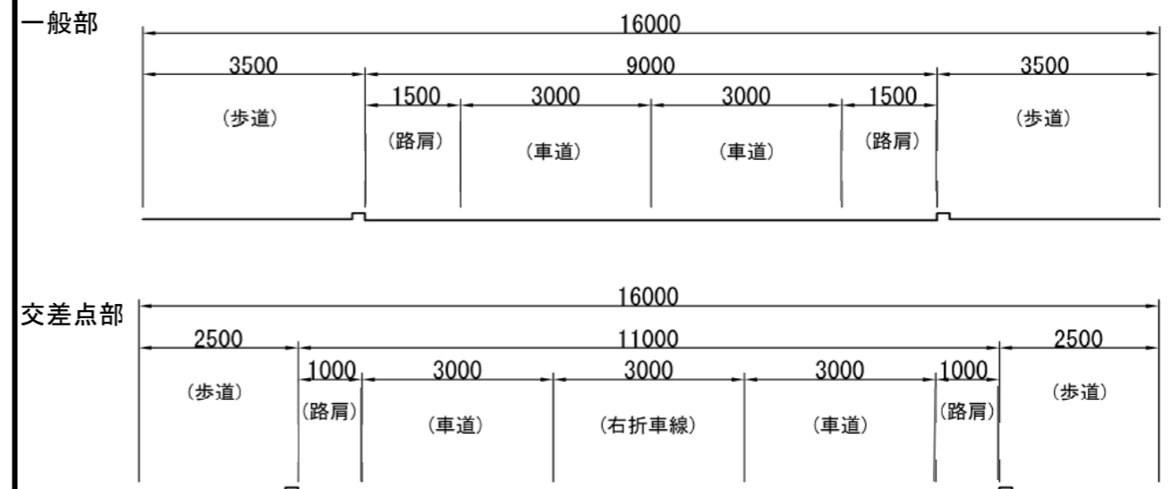
標準断面図
