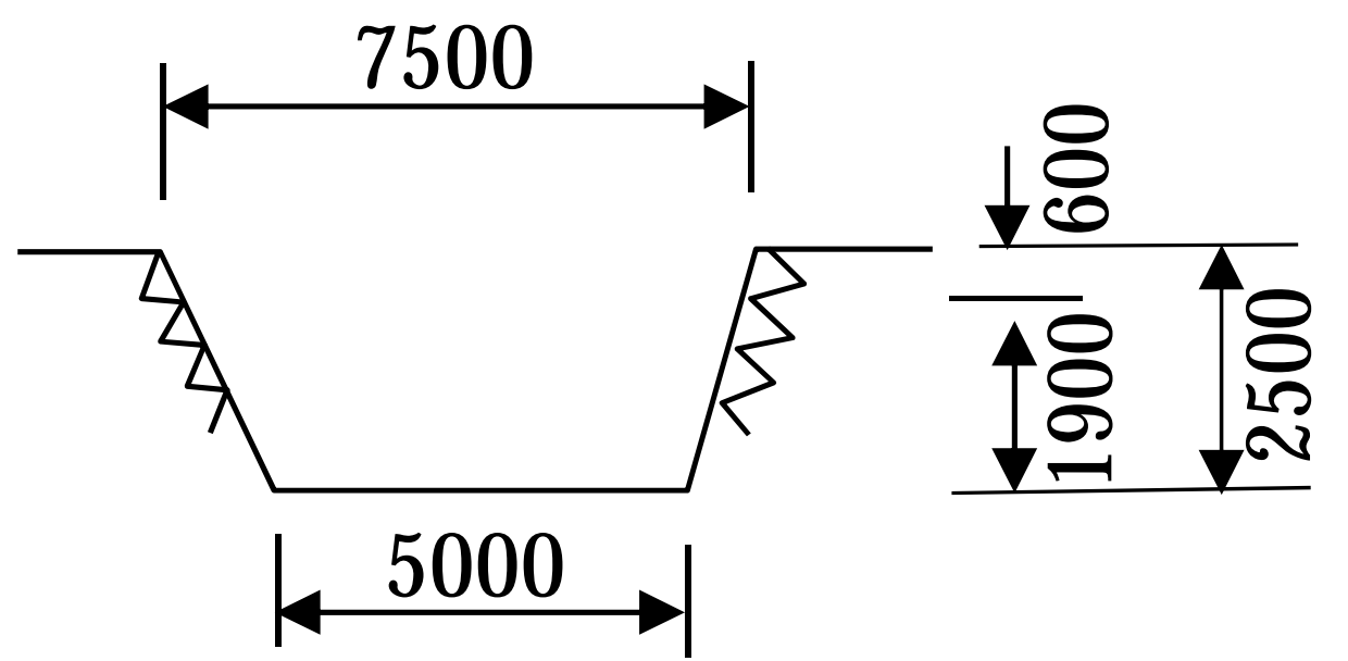
標準断面図
