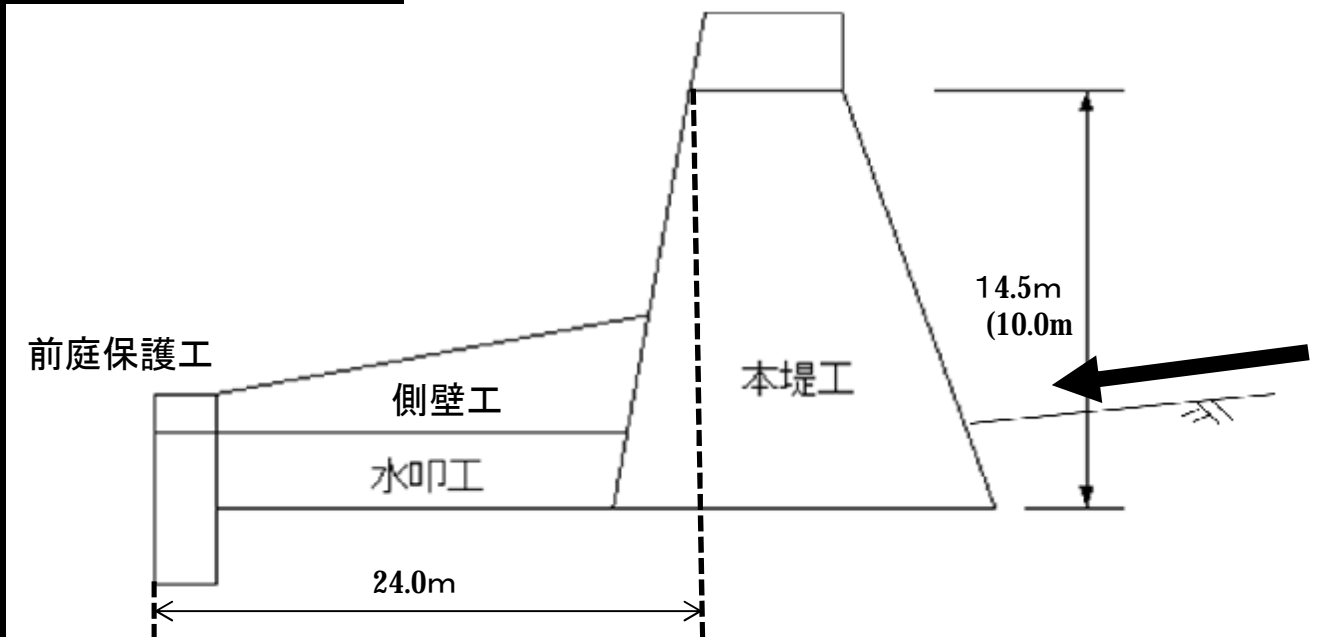
標準断面図
