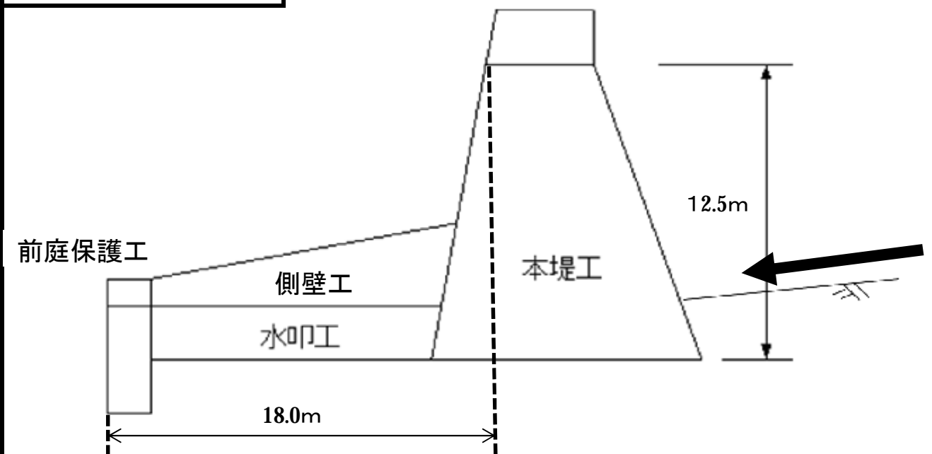
標準断面図
