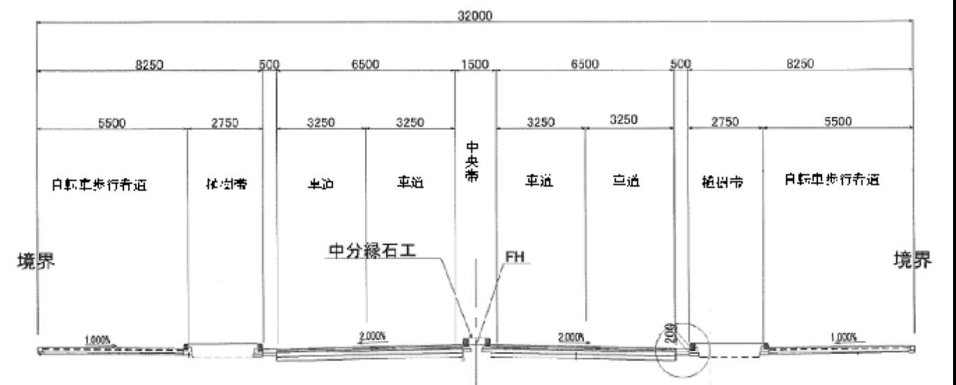
標準断面図
