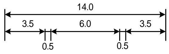
標準横断面図
