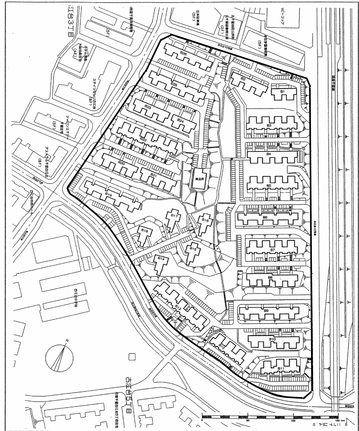
現敷地現況図
