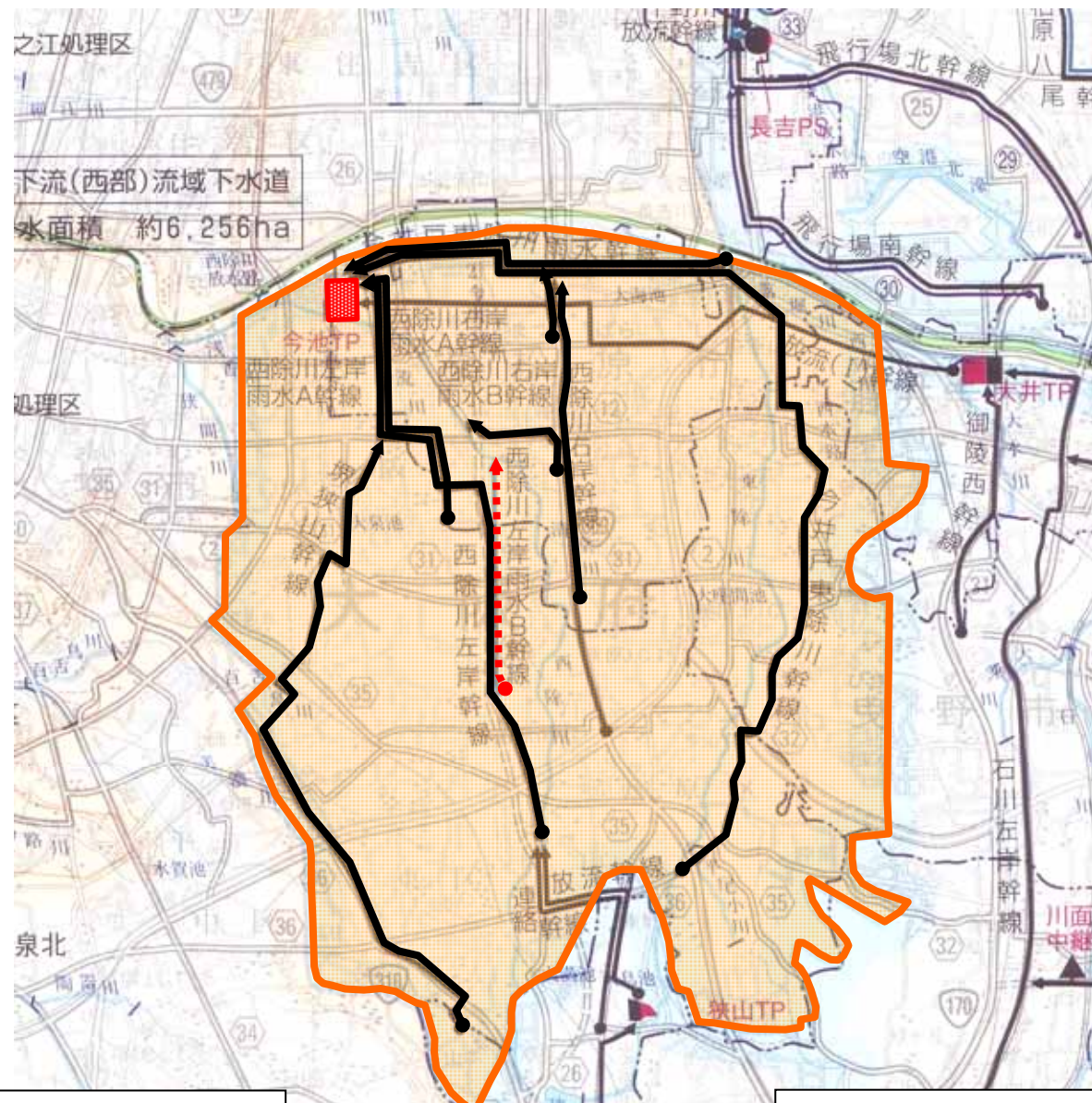
事業箇所図
