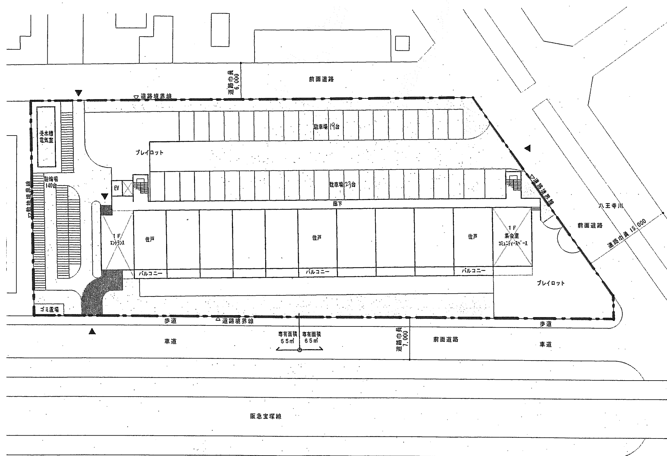
計 画 図
