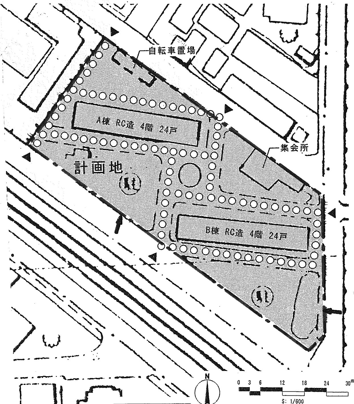
現況図
