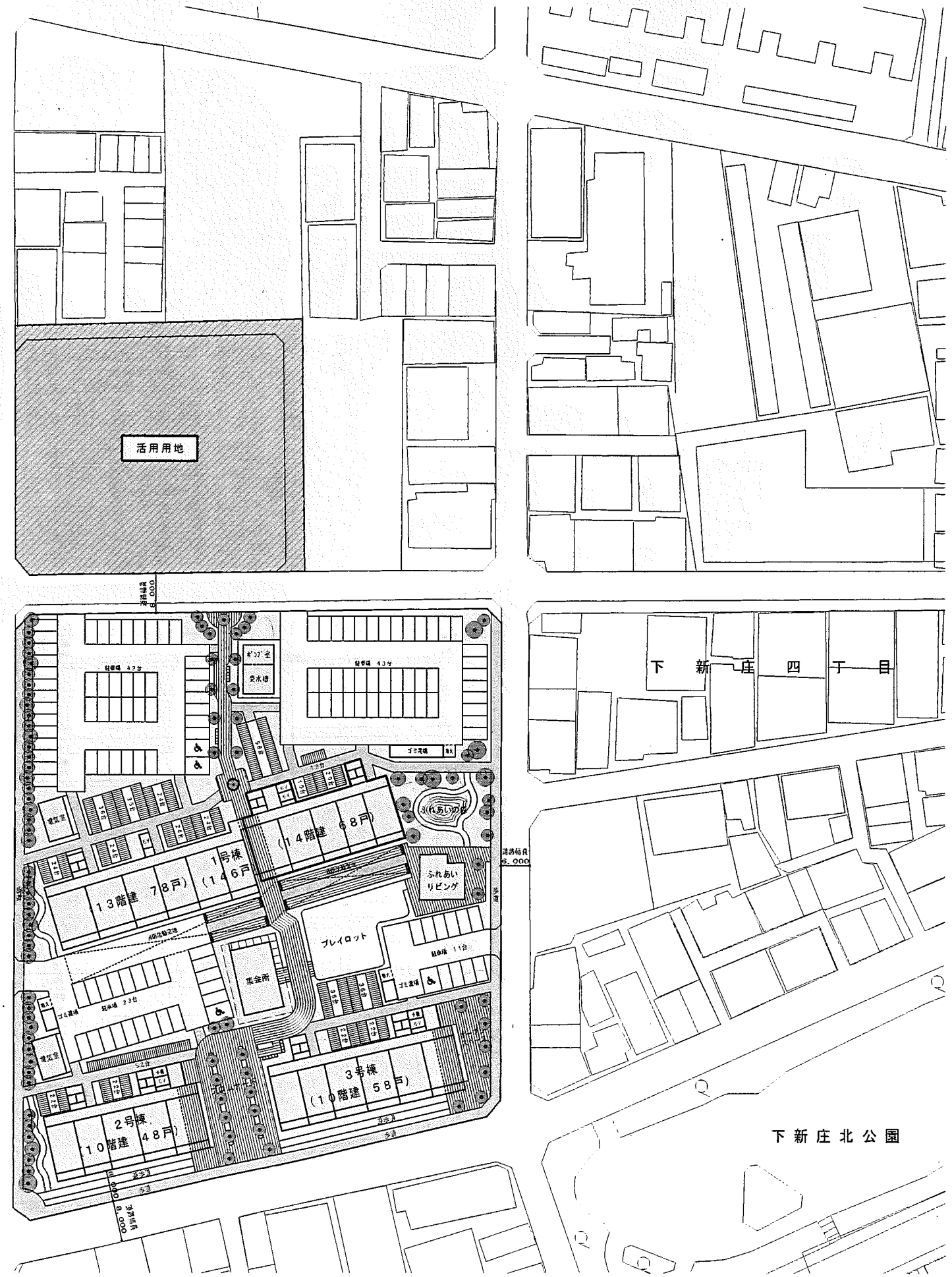
計画図
