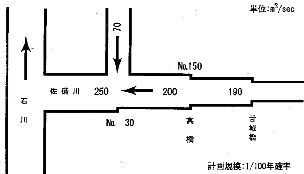
流量配分図
