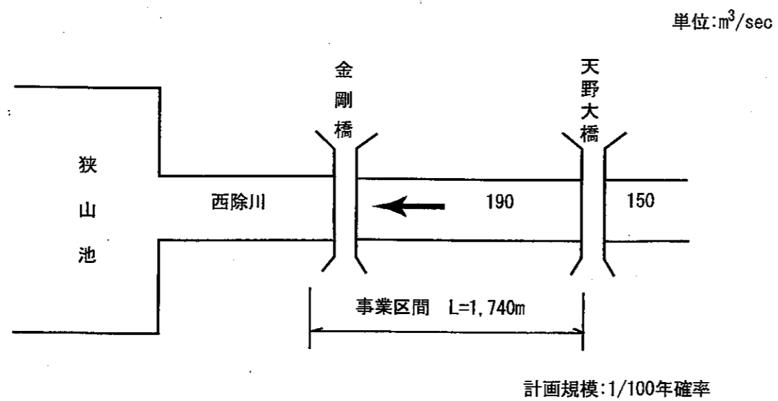
流量配分図
