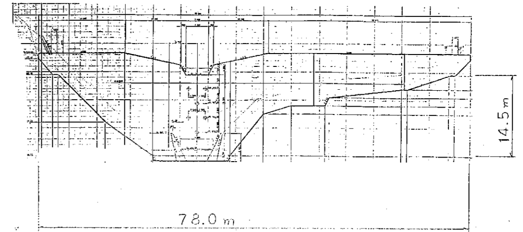
正面図
