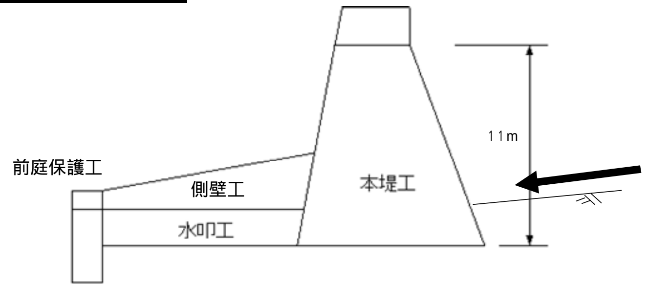
標準断面図
