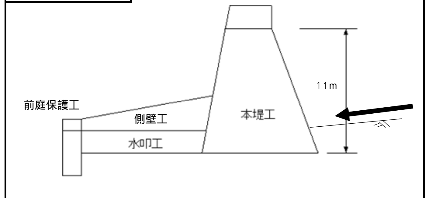
標準断面図
