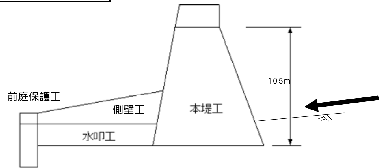
標準断面図
