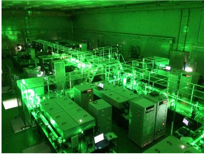
関西研の極短パルス高強度レーザー装置 (J-KAREN)
