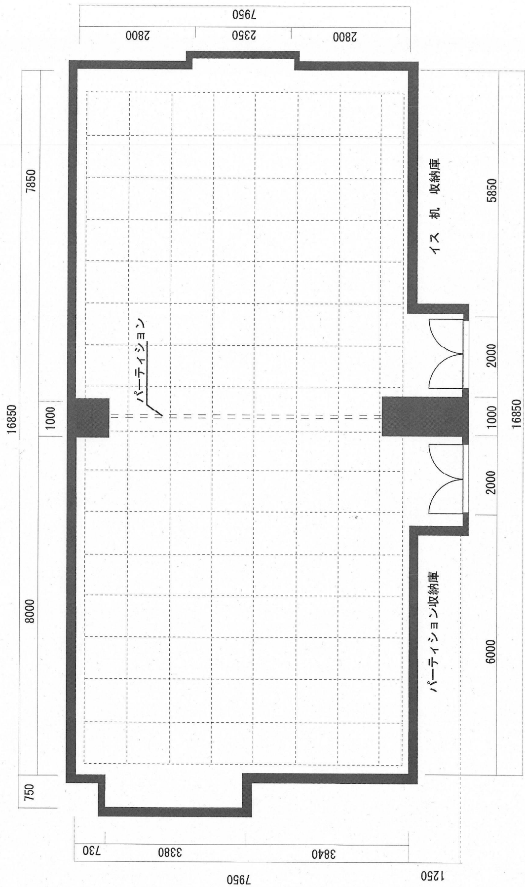
大阪府立中央図書館 大会議室 平面図 138㎡ 単位=mm
