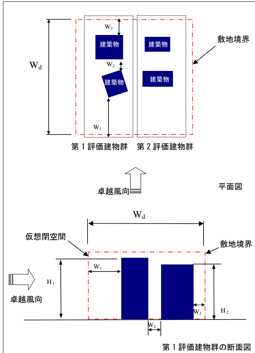
図16 同一敷地内に複数棟がある場合の評価方法
