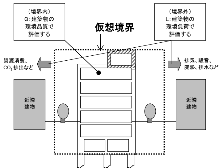
図Ⅲ.1.5 仮想閉空間の概念に基づく「Q 建築物の環境品質」と「L 建築物の環境負荷」の評価分野の区分
