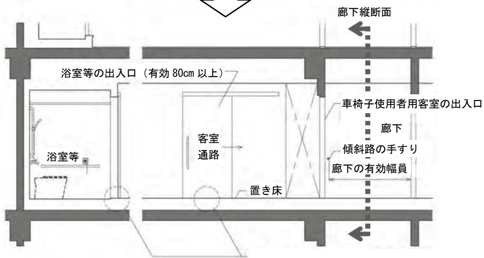
廊下縦断面
