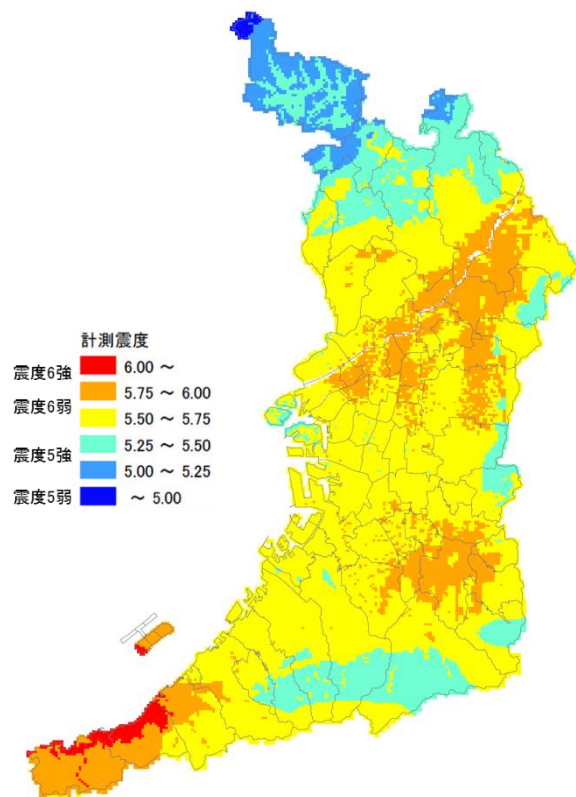
【計測震度】
