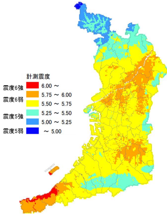
【計測震度】
