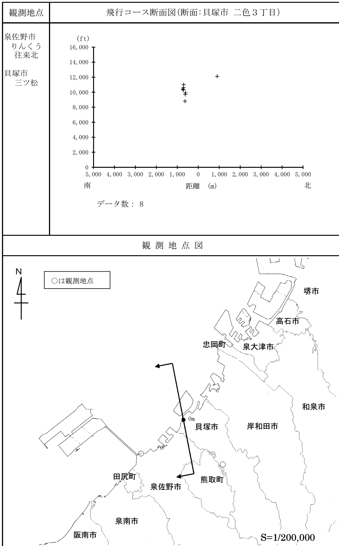
図3-9(2) 航空機飛行経路・高度の観測結果(着陸)
