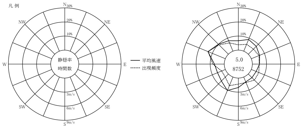
図(1)-1-1 気象(風向・風速)の観測結果
