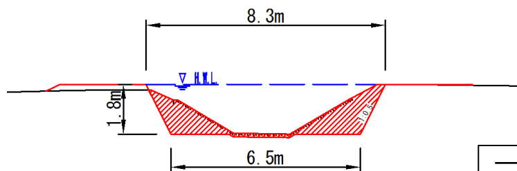
図-2.14 整備断面例(7.20km付近)
