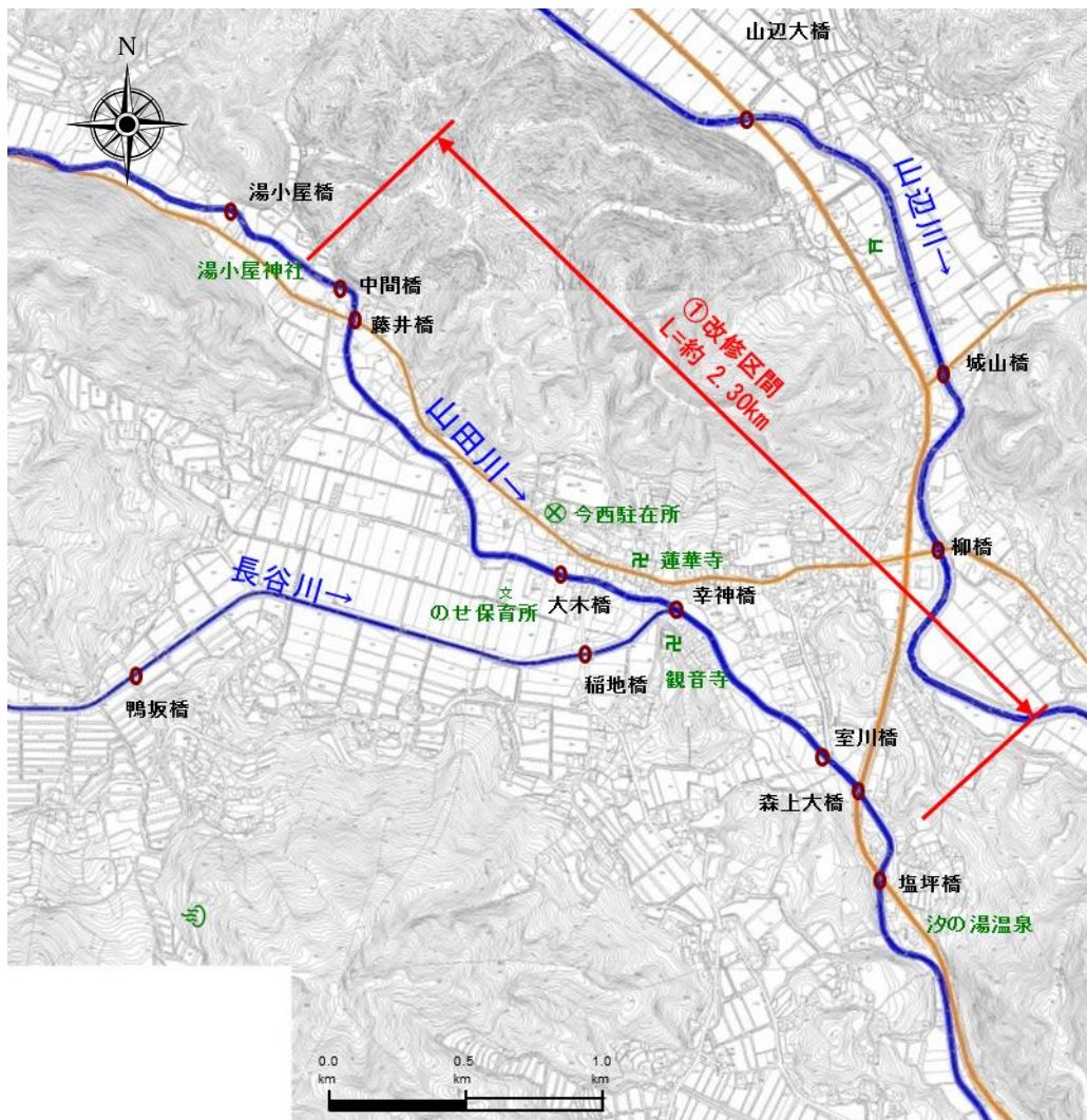
図-2.6 整備対象区間平面図(山田川)
