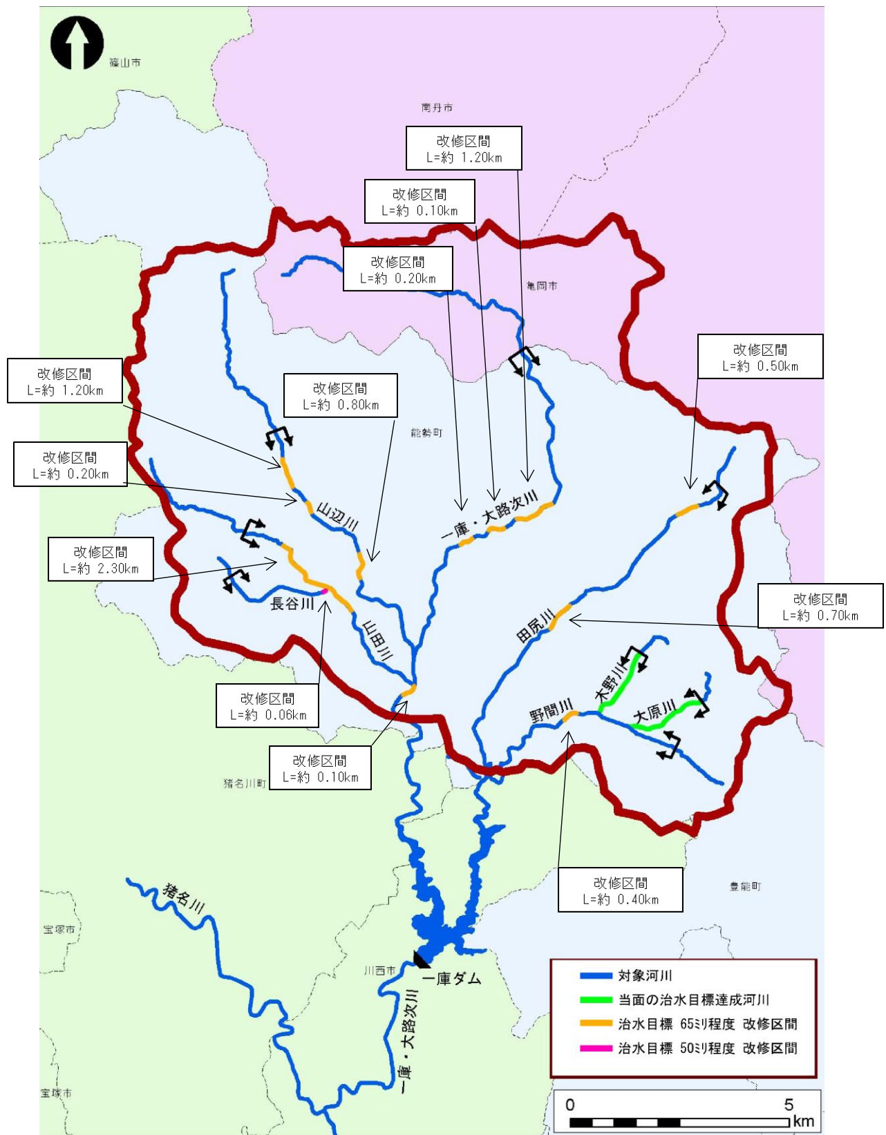
図-2.1 整備対象区間平面図
