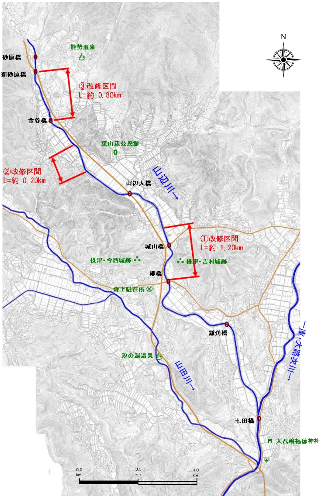
図-2.12 整備対象区間平面図(山辺川)
