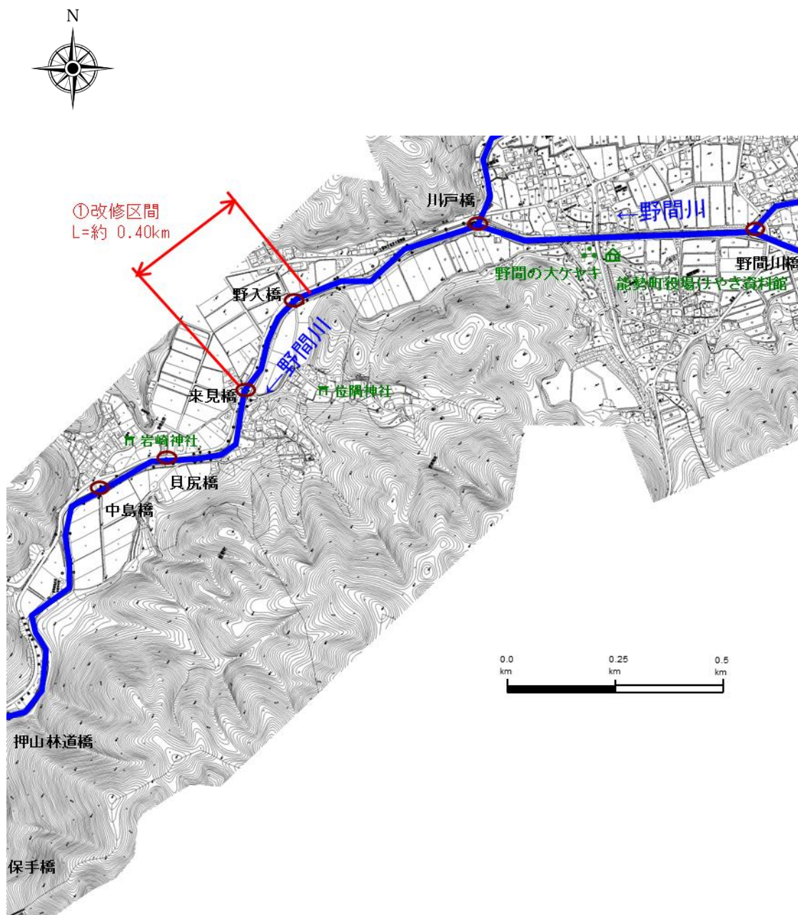
図-2.17 整備対象区間平面図(野間川)
