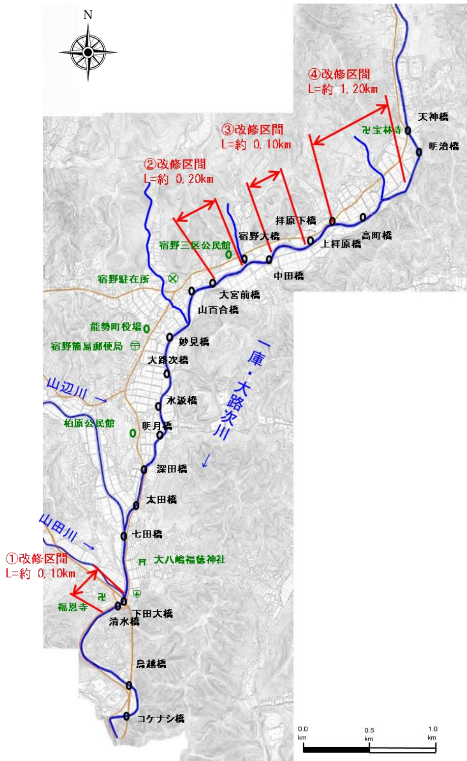
図-2.4 整備対象区間平面図(一庫・大路次川)
