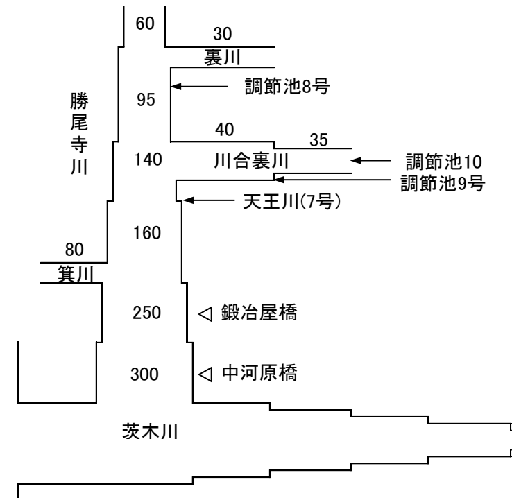
勝尾寺川流量配分図
