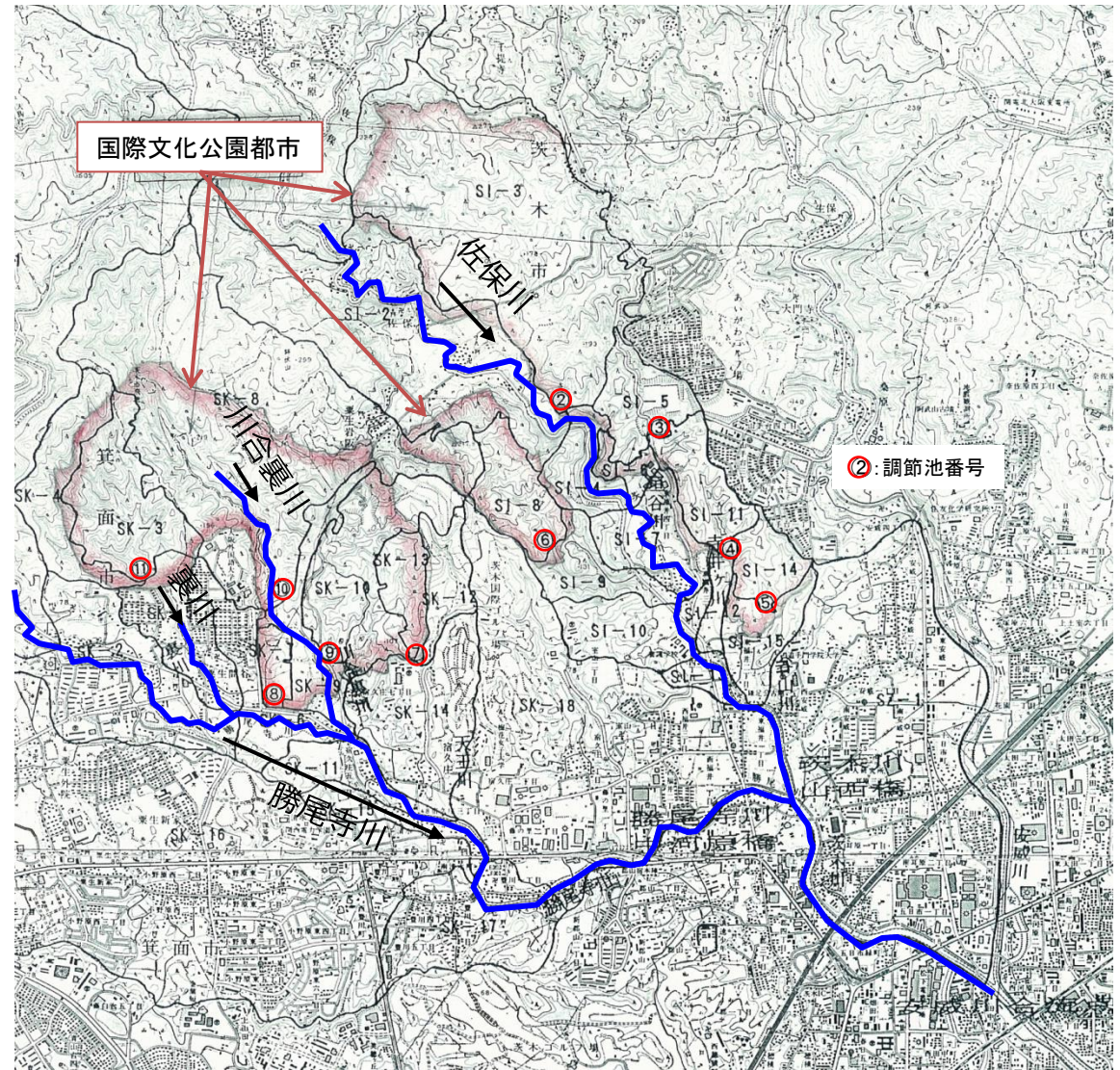
調節池の配置と調節池諸元（茨木川全体計画（平成7年）より）
