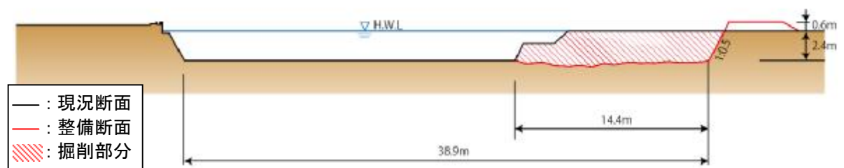
図- 2.4 整備断面例 (10.5km 付近)
