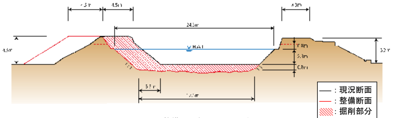
図-2.14 整備断面例(0.6km 付近)
