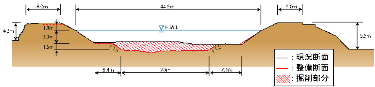
図- 2.3 整備断面例 (3.7km 付近)
