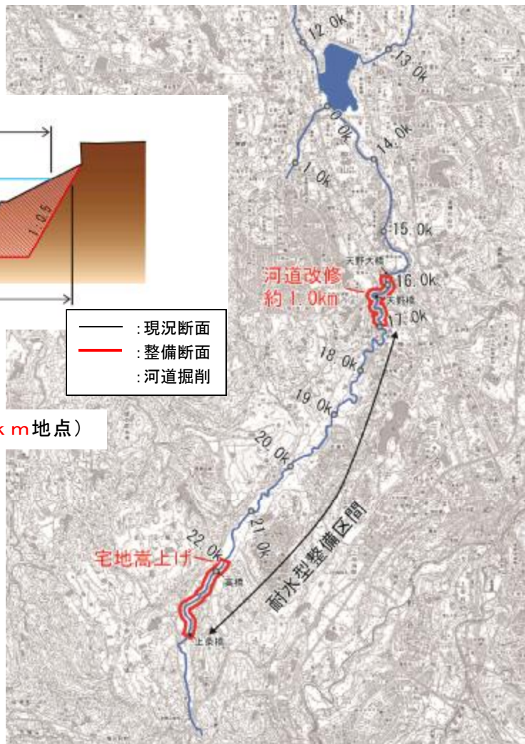
図 2.4 整備対象区間平面図
