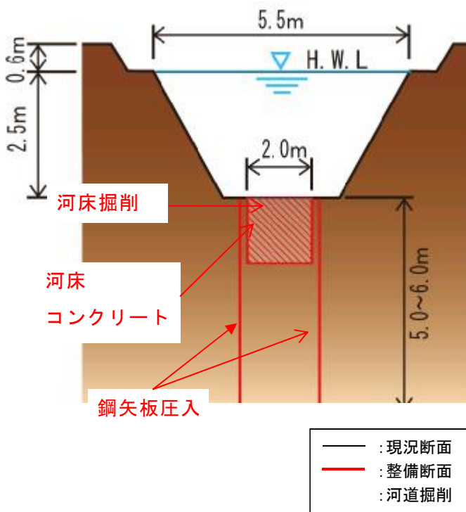
図 2.9 整備断面例 (1.6 km地点)
