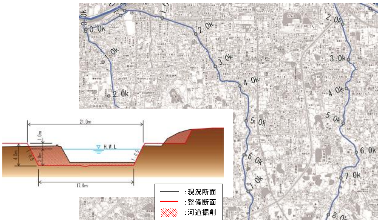
図 2.3 整備断面例（10.0 km地点）
