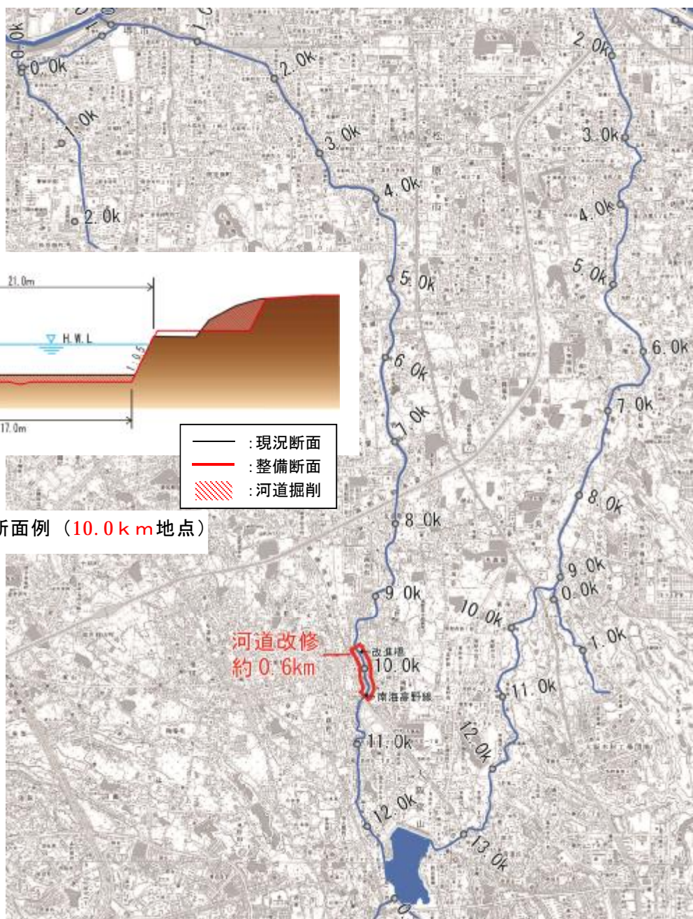
図 2.2 整備対象区間平面図
