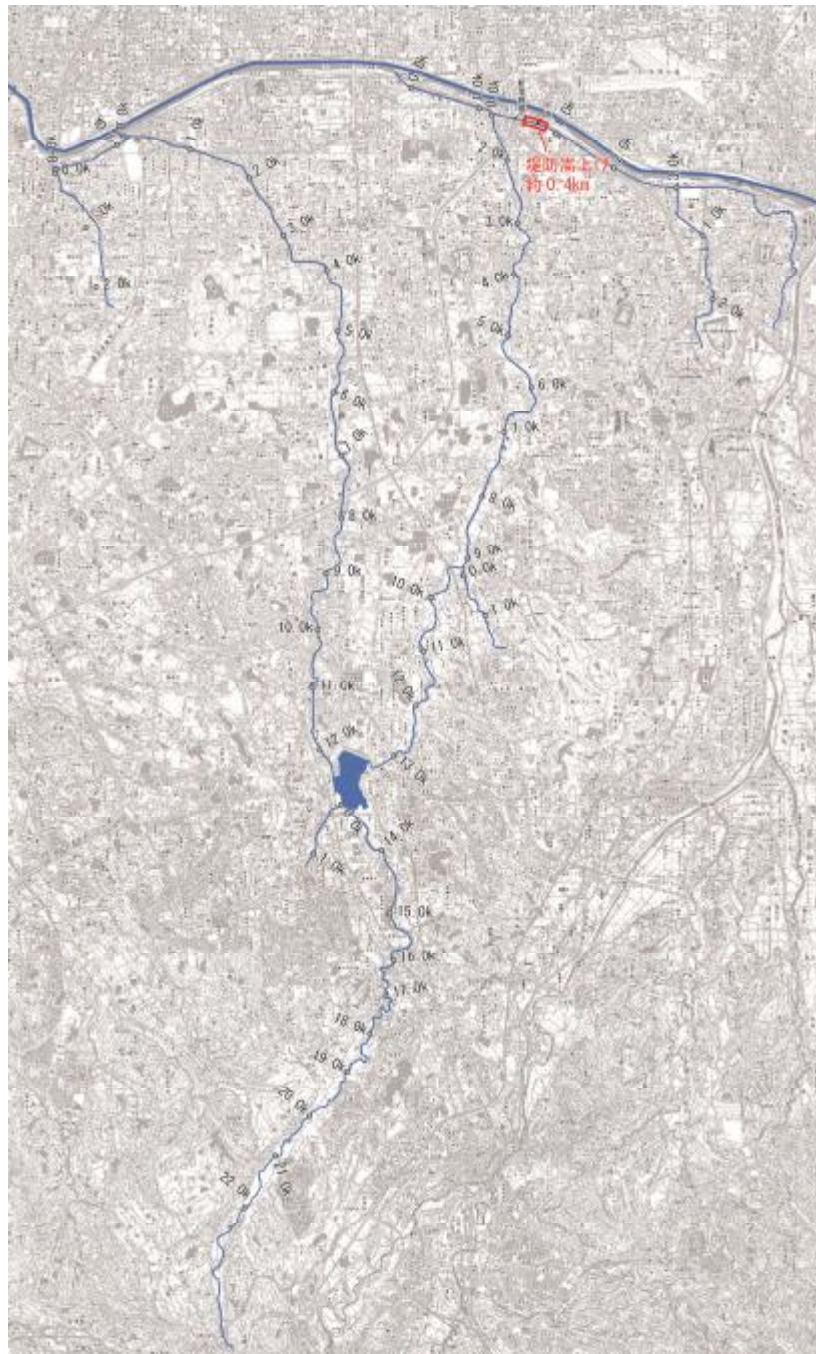
図 2.10 整備対象区間平面図
