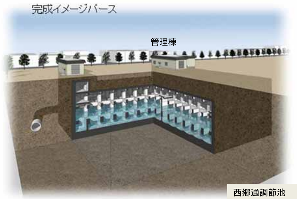
図 2.12 さいごうどおり 西郷通調節池完成イメージ
