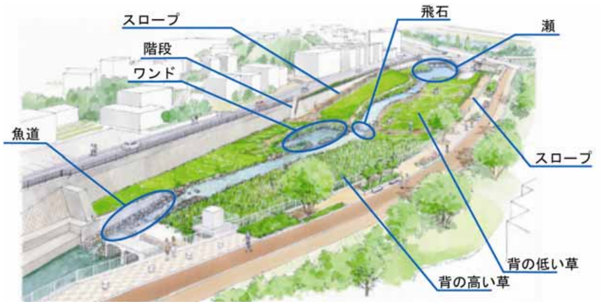
図 2.14 打上川治水緑地下流の親水空間整備イメージ
