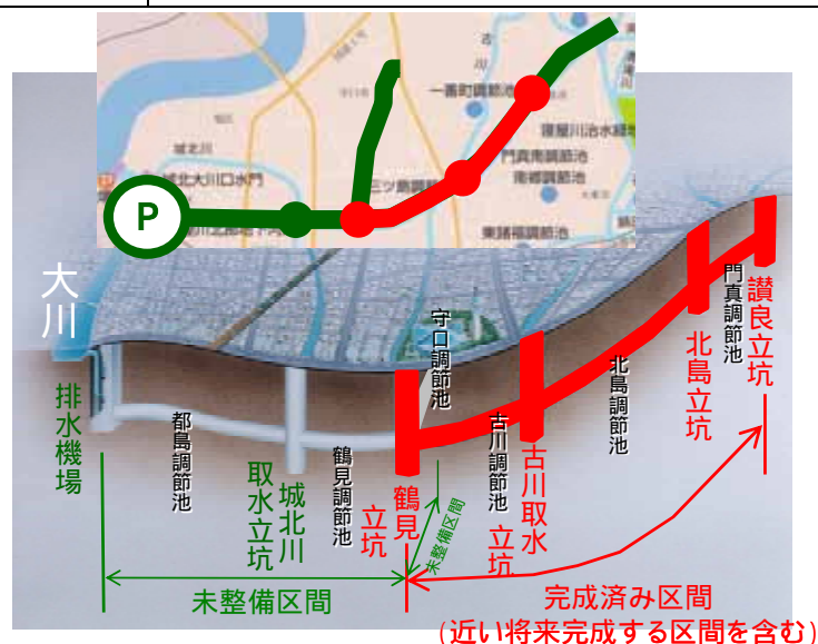
図 2.10 寝屋川北部地下河川完成イメージ
