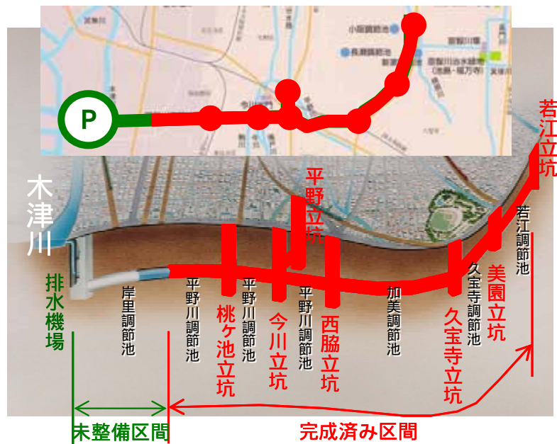
図 2.11 寝屋川南部地下河川完成イメージ
