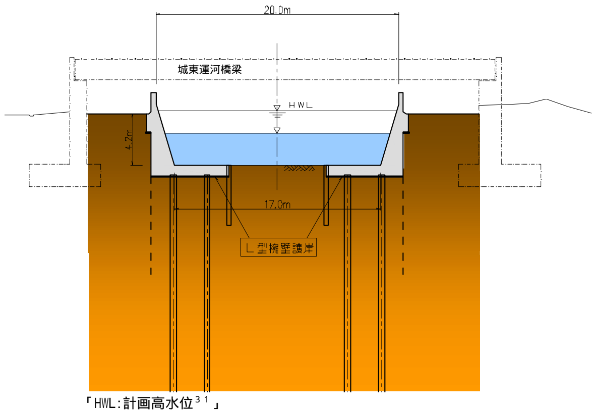
図 2.2 JR 学研都市線及び大阪外環状鉄道 城東運河橋梁部 じょうとう 護岸 標準断面図
