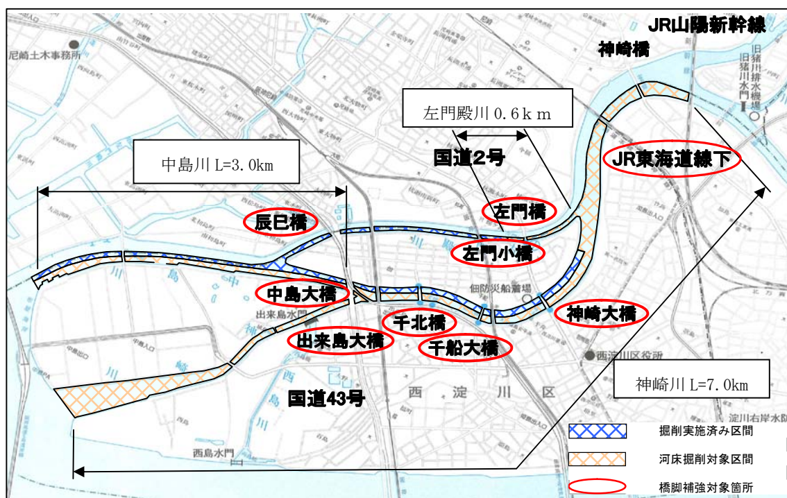
図 河床掘削・橋脚補強対象箇所
