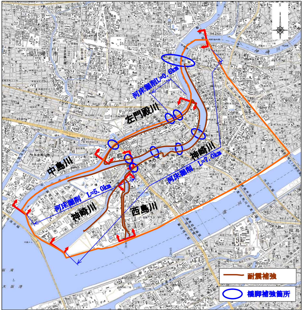
図 整備対象区間位置図
