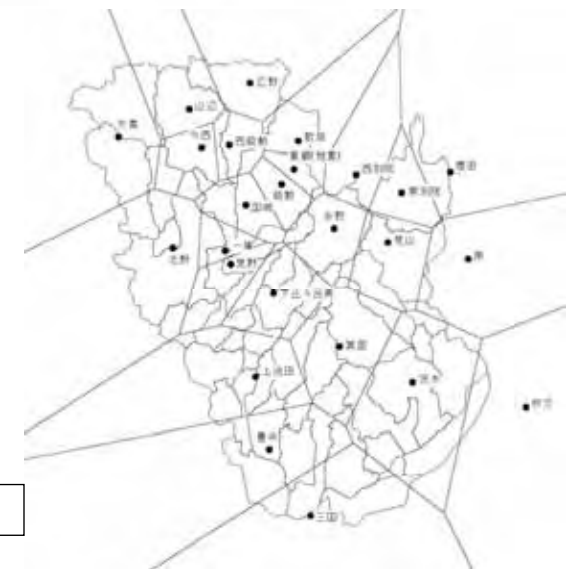
図-2.9 日雨量ティーセン分割図の例
