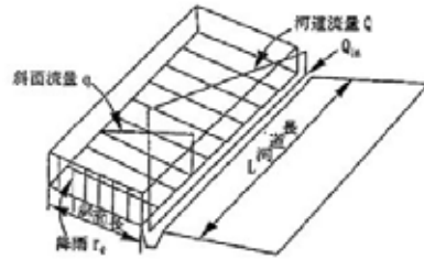
図一 特性曲線法の流域のモデル
