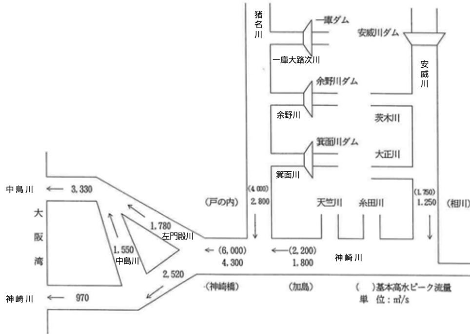
図-2.4 基本高水ピーク流量と計画高水流量 流量配分図
