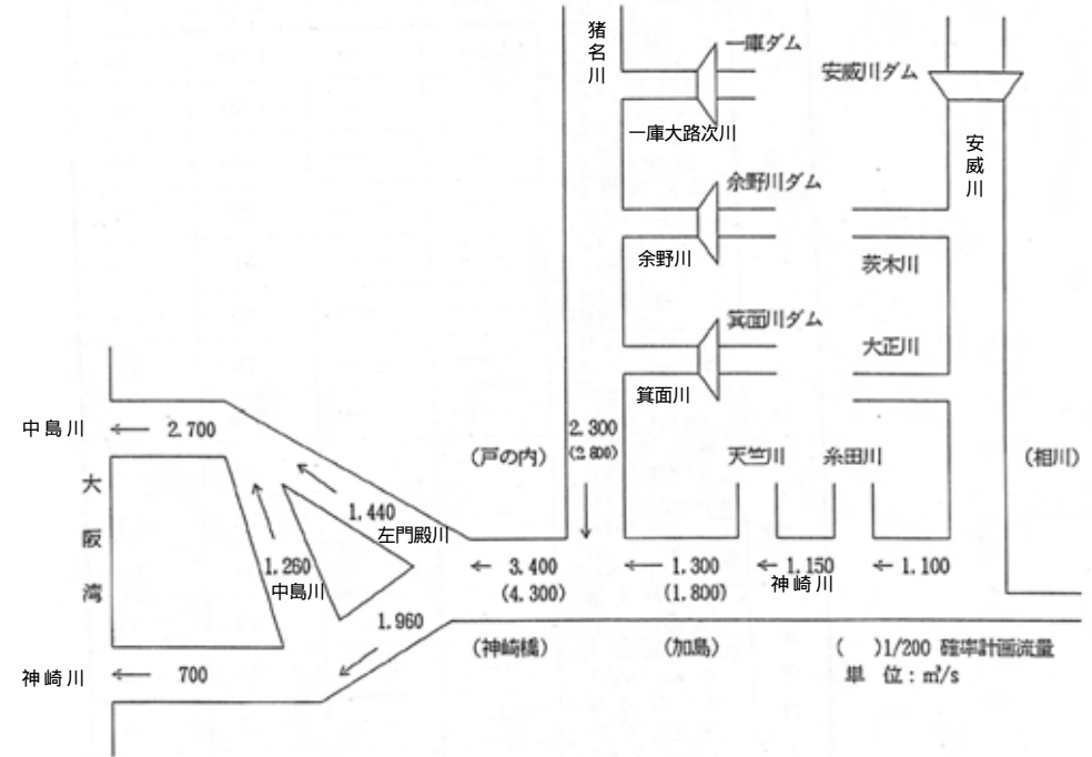
図-2.5 神崎川 1/40 確率計画流量配分図
