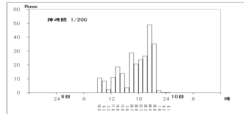
図-2.3 昭和42年7月型 降雨ハイエトグラフ
