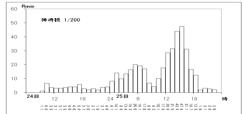
図-2.2 昭和28年9月型 降雨ハイエトグラフ
