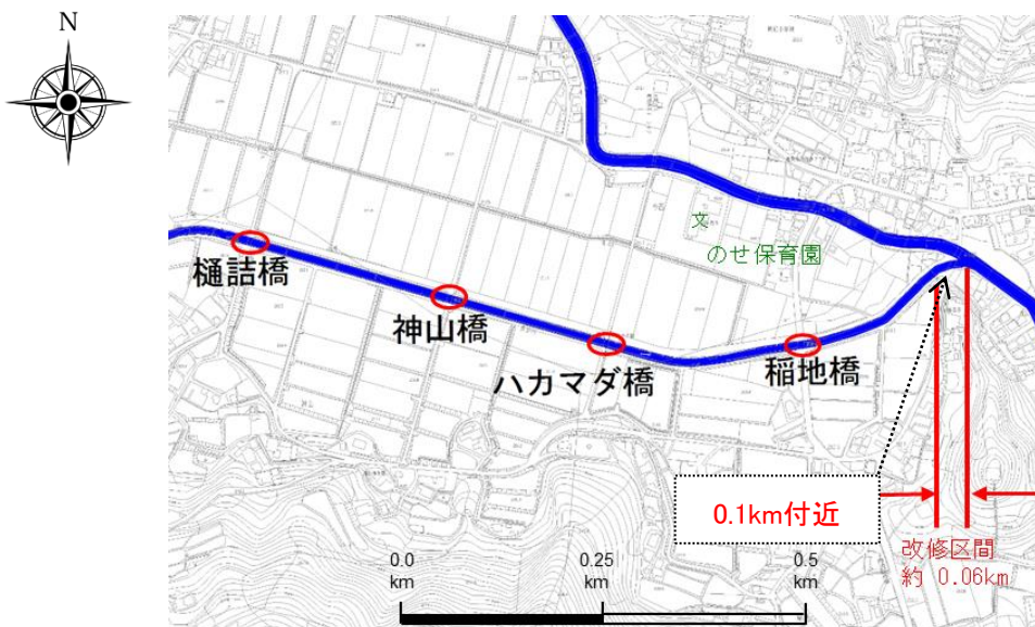
図-2.8 整備対象区間平面図(長谷川)
