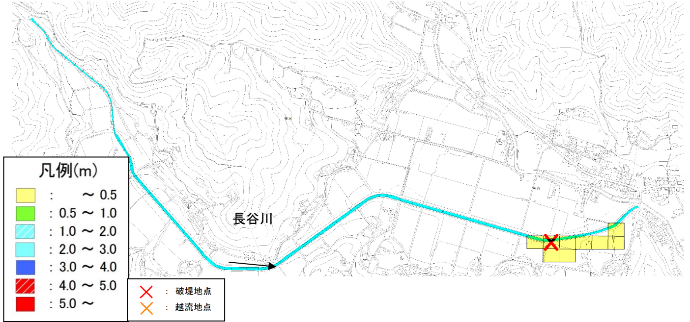
図-3.3 長谷川 洪水リスク表示図
