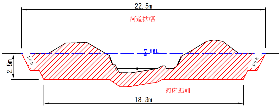
図-2.13 整備断面例(4.1km付近)
