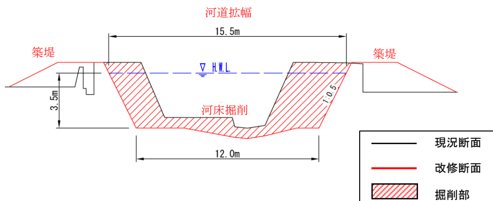
図-2.5 整備断面例(2.7km 付近)
