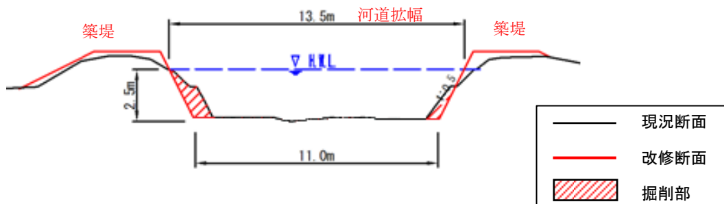
図-2.11 整備断面例(4.3km付近)
