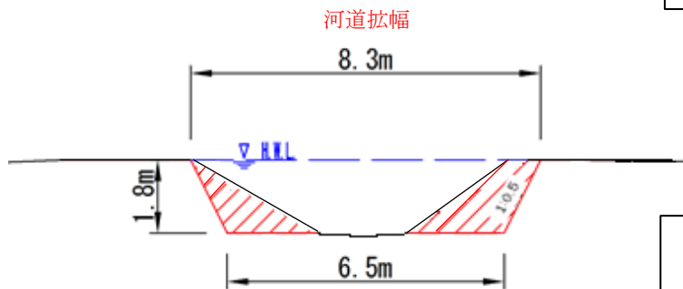
図-2.14 整備断面例(7.2km付近)
