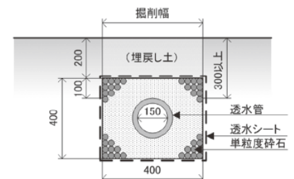
図26 浸透レンチの例
