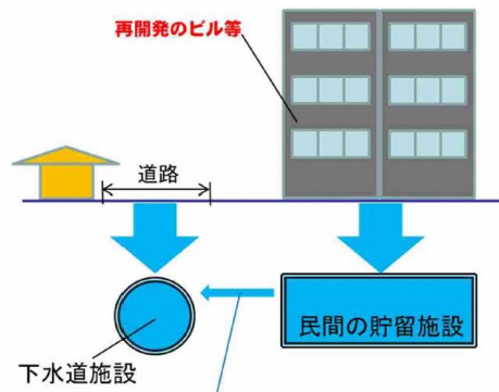
寝屋川流域における浸水対策
