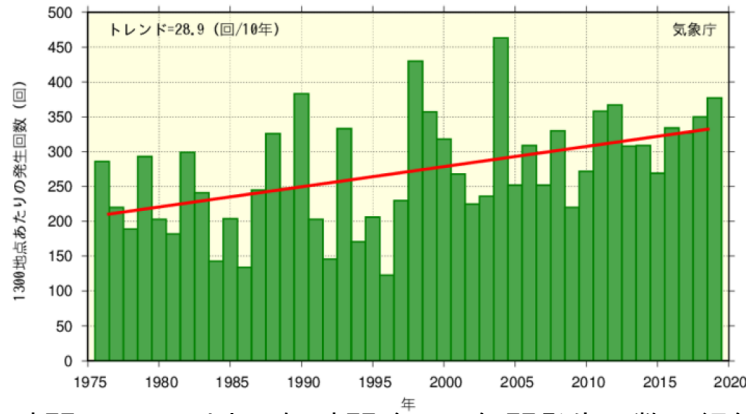
国内の1時間50mm以上の短時間強雨の年間発生回数の経年変化 出典:日本の気候変動(2020年12月文部科学省、気象庁) 「棒グラフ(緑)は各年の年間発生回数(全国のアメダスによる観測値を1,300地点あたりに換算した値)。直線(赤)は長期変化傾向(この期間の平均的な変化傾向)を表します。」
