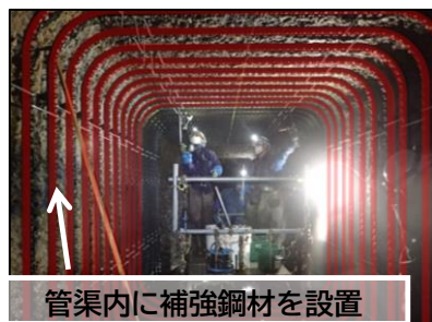
管きよ耐震化の例
