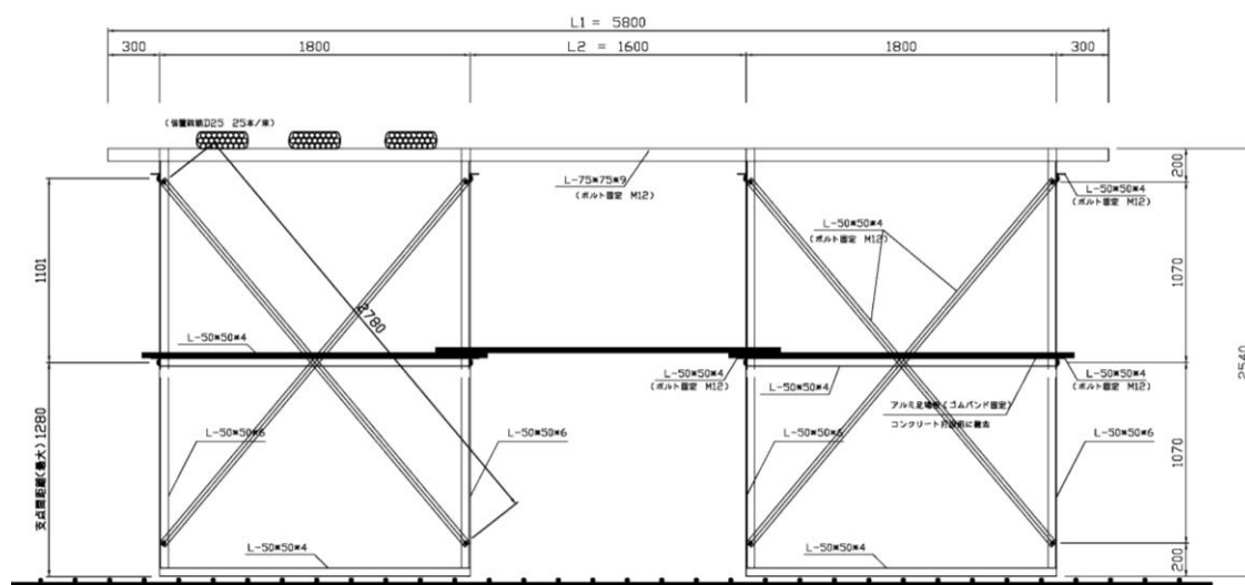
A-A 断面図
