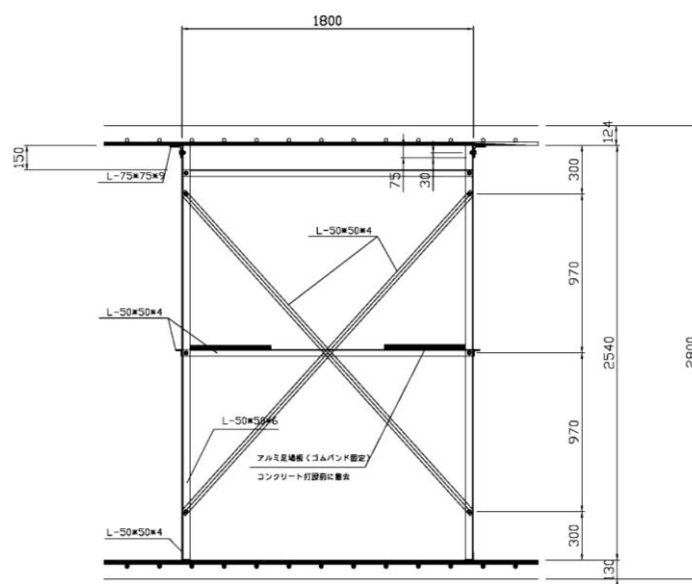
B-B 断面図
