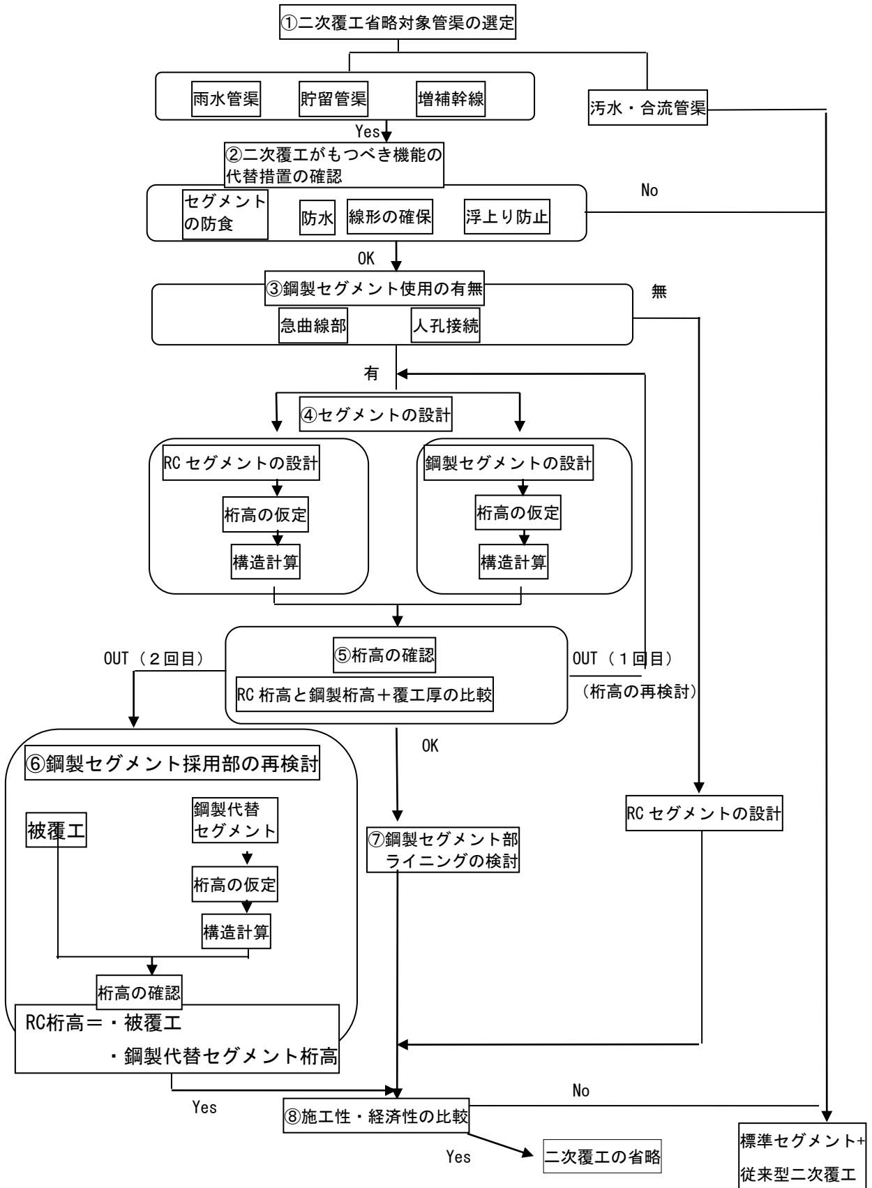
図 6-1-7 フロー図
