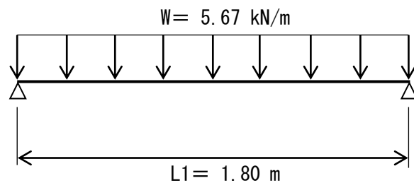
図 2-3-5 単純梁
