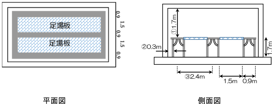
図 8-1-2 天井、壁面施工の場合の概略図
