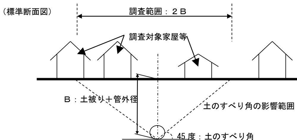
図 1-2-3 標準断面図
