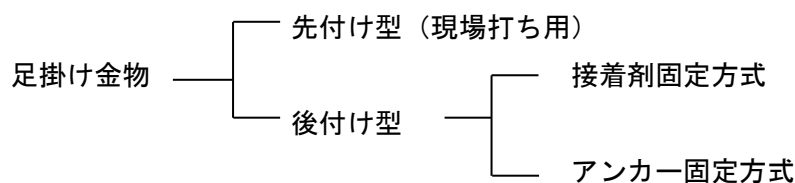
図 4-2-2 足掛け金物の施工方式
