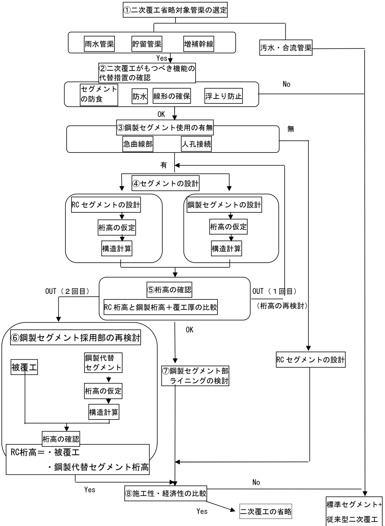
図 6-1-7 フロー図
