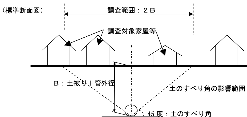
図 1-2-3 標準断面図
