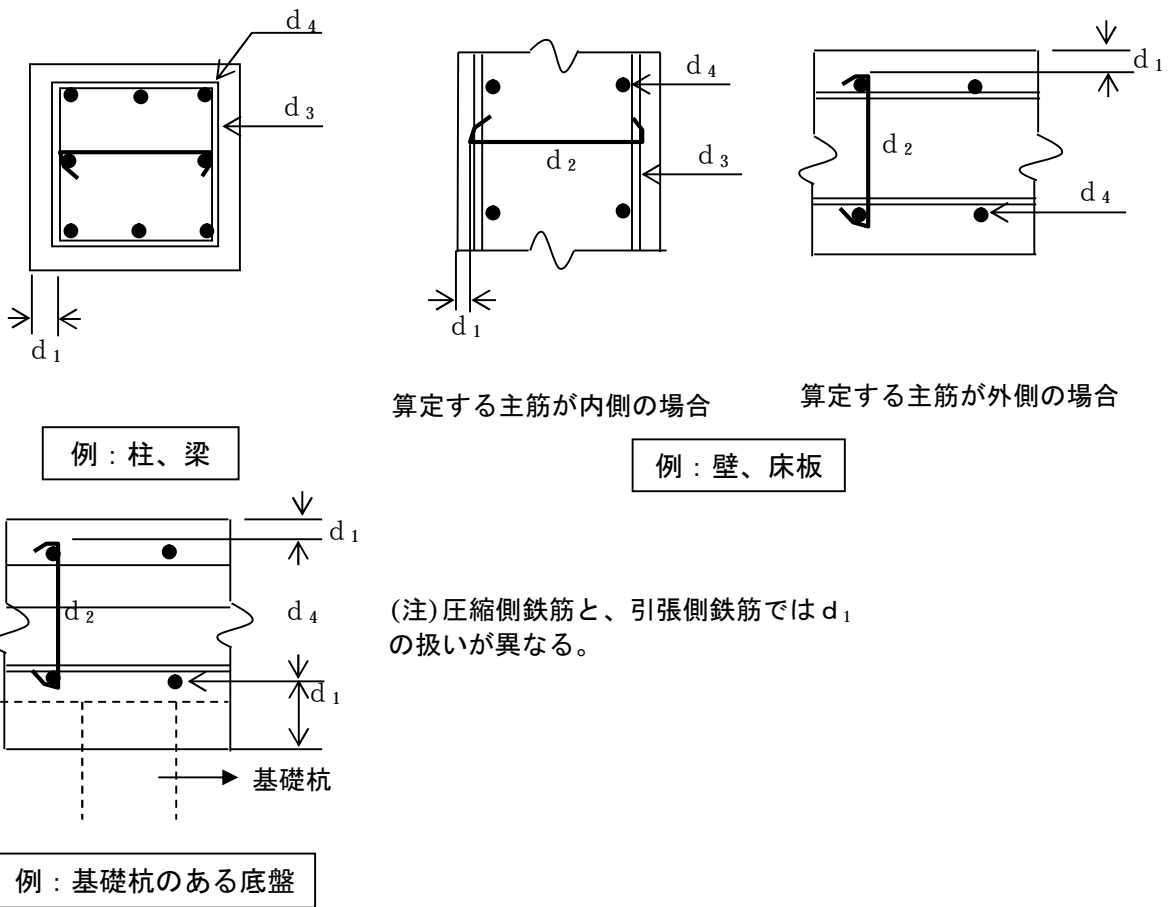
図 2-3-1 最小かぶり
