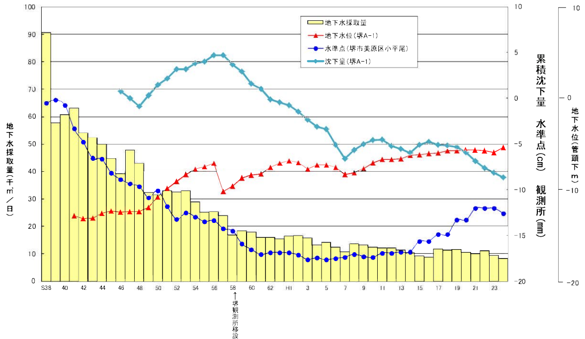
図2-7 地下水採取量と地下水位・累積沈下量の相関(堺市)
