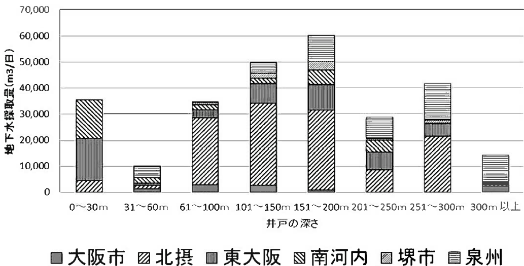
図2-9 井戸深度別地下水採取量
