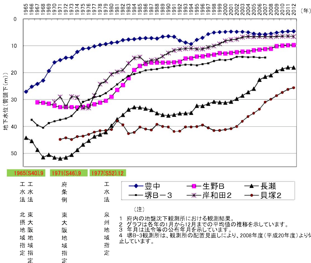
図2-2 地下水位の推移
