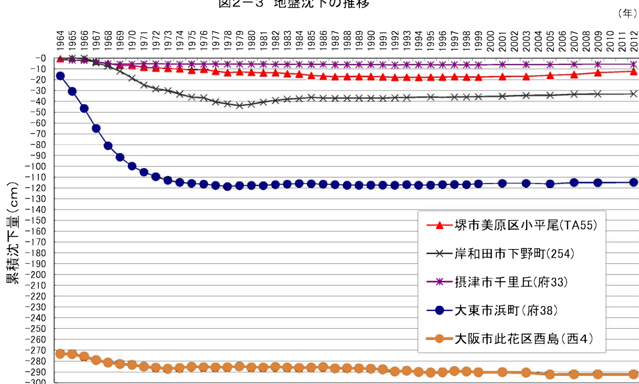
図2-3 地盤沈下の推移
