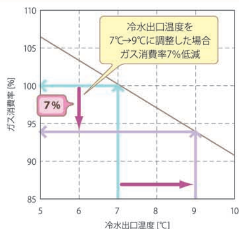
【冷水出口温度とガス消費率(吸収式冷温水機)】 出典:2012ビル省エネ手帳(財)省エネルギーセンター
