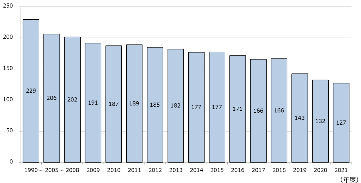
図 17 廃棄物部門における二酸化炭素排出量の推移
