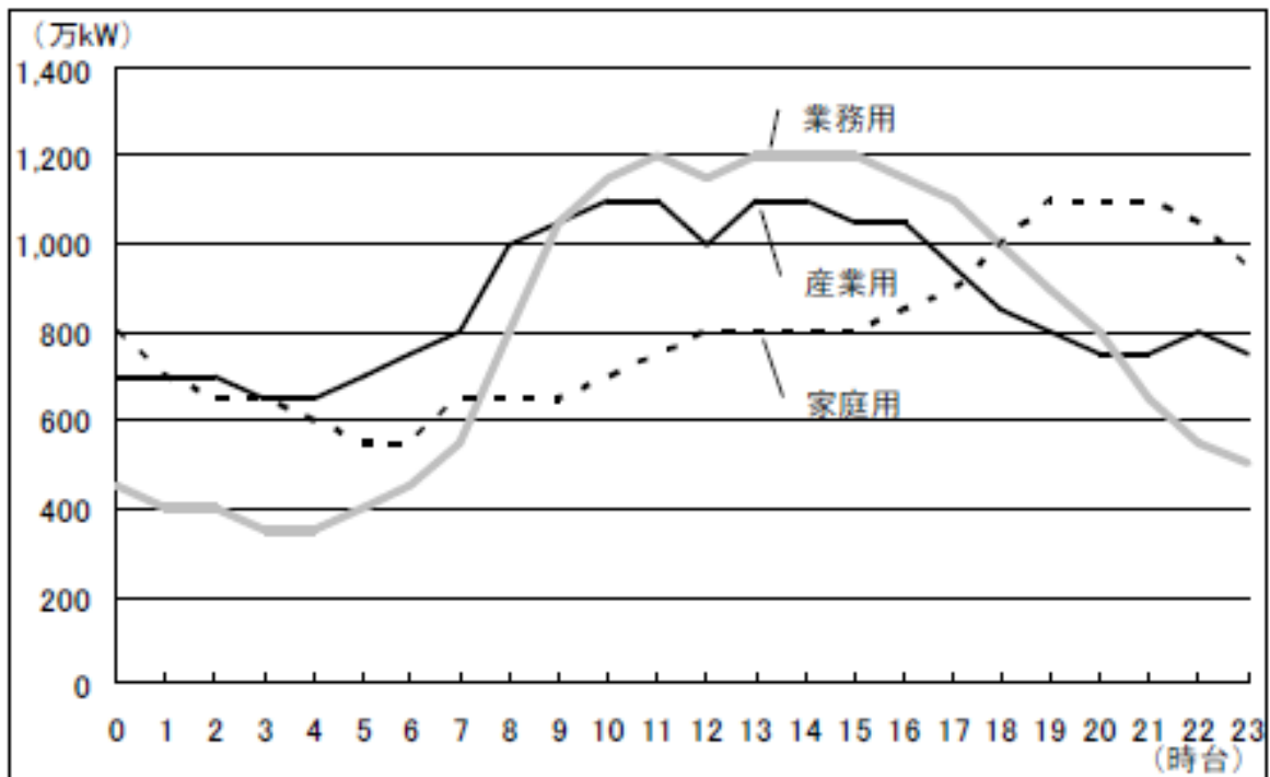
図26 夏期のピーク発生日(2010年8月19日)における電力需要曲線(推計値)
