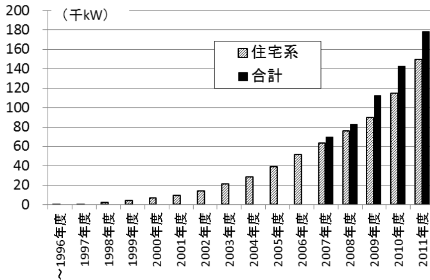
図46 太陽光発電の導入実績の推移
