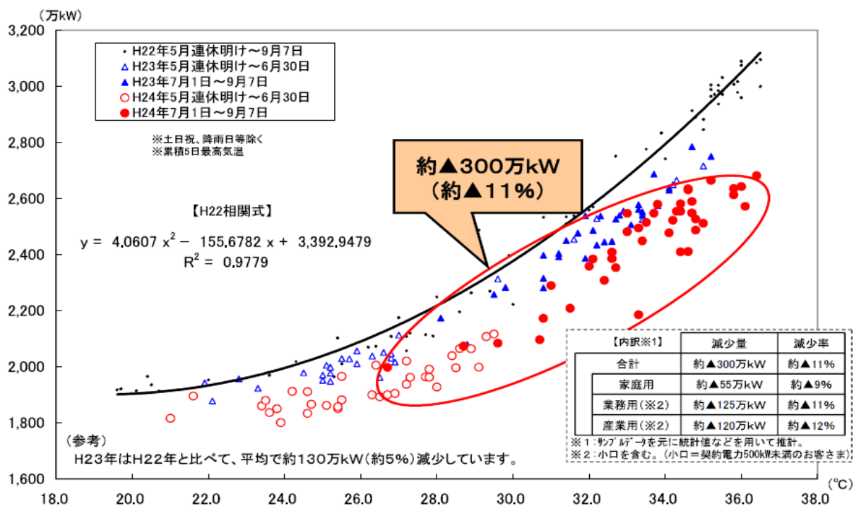
図 36 夏期の14～15時の使用電力の比較 (対2010年)
