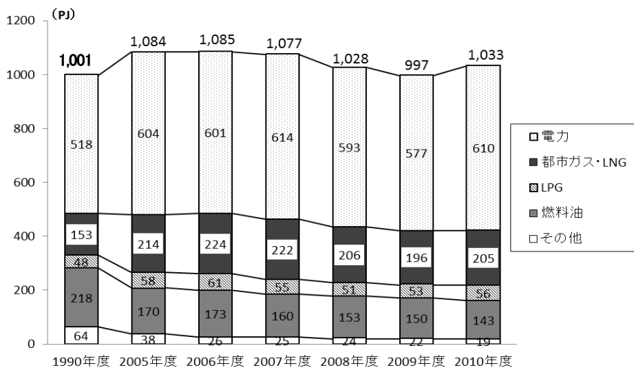
図 5 府域の燃料種別エネルギー消費量(一次エネルギーベース)の推移
