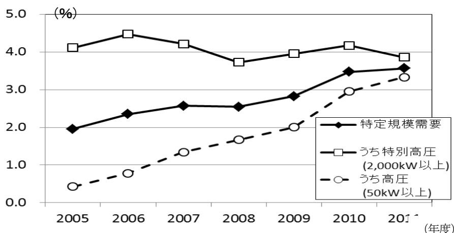
図 44 新電力（PPS）の全体販売電力量に占めるシェア（全国）
