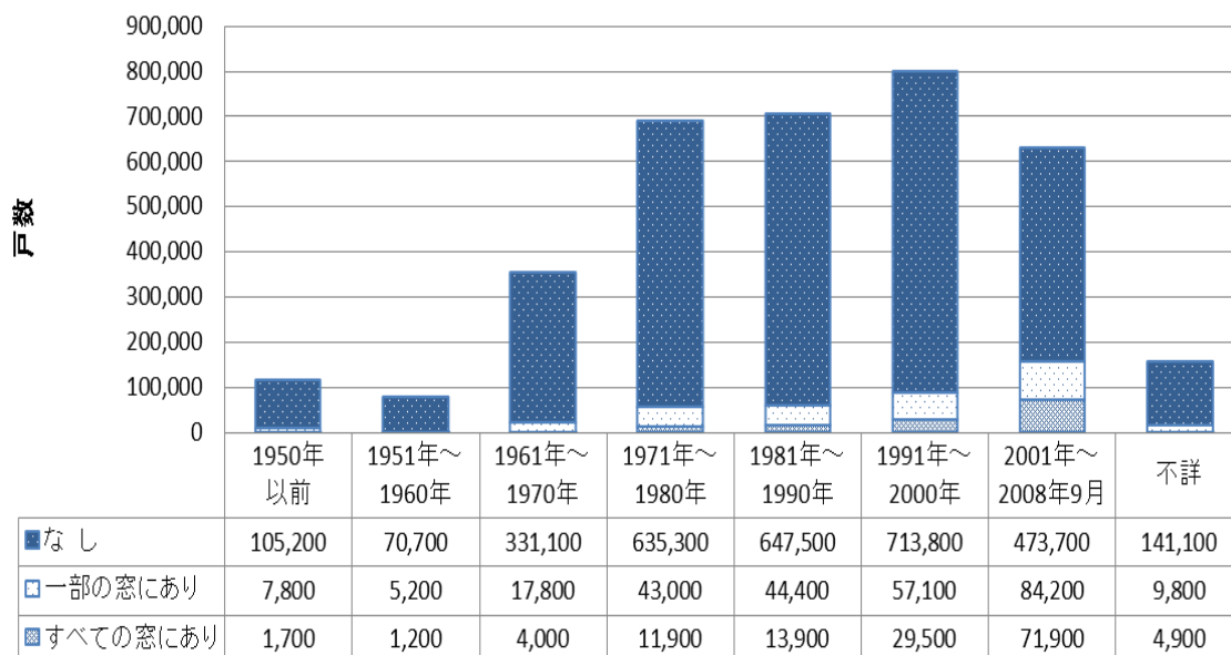
図 17 府域の住宅に二重サッシ又は複層ガラスを設置している戸数（建築年別）
