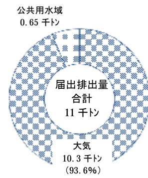
2012年度の府域における化学物質の届出排出量 府域における化学物質排出量のうち9割以上が大気への排出となっています。
