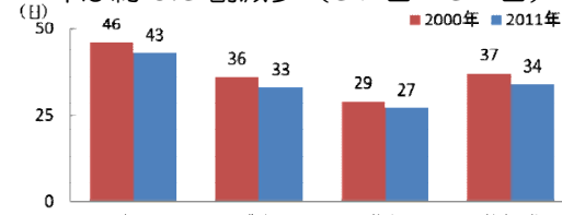
大阪府域における熱帯夜数の推移 (2000年、2011年と各5年移動平均値)
