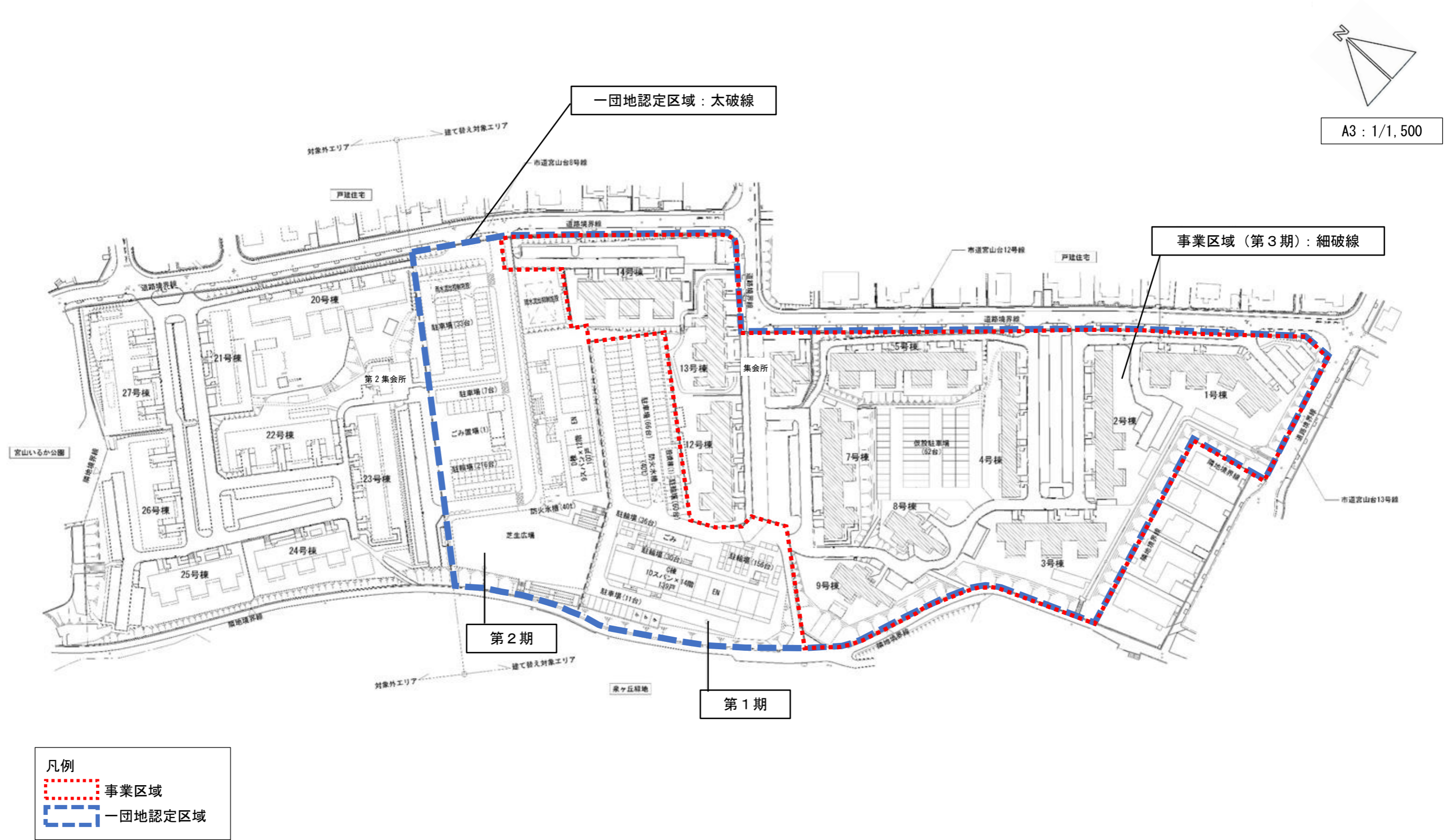
添付図8 一団地認定区域図（府営住宅整備用地）
