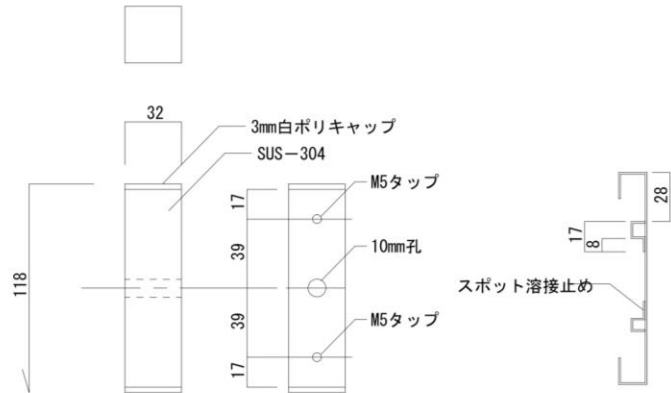
■詳細図 S=1 : 3
