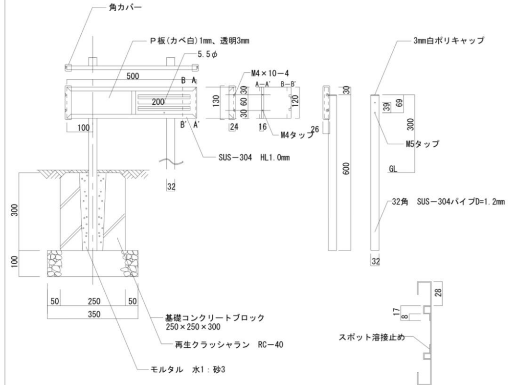
■詳細図 S=1 : 3
