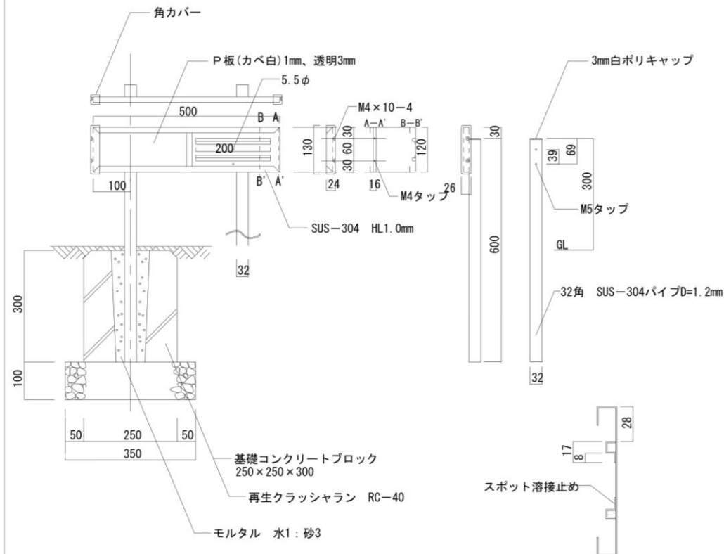
■詳細図 S=1 : 3
