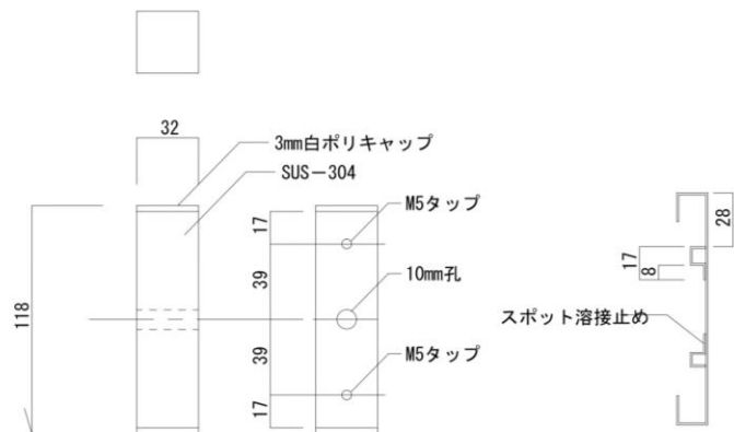
■詳細図 S=1 : 3
