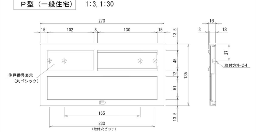
添付図 10 各部詳細図 (表札 : 住戸入口)
