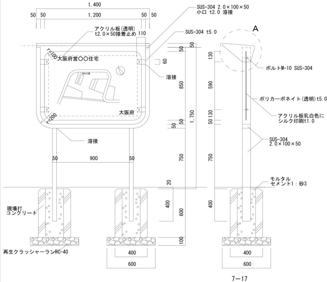
添付図 10 各部詳細図 (団地案内板)
