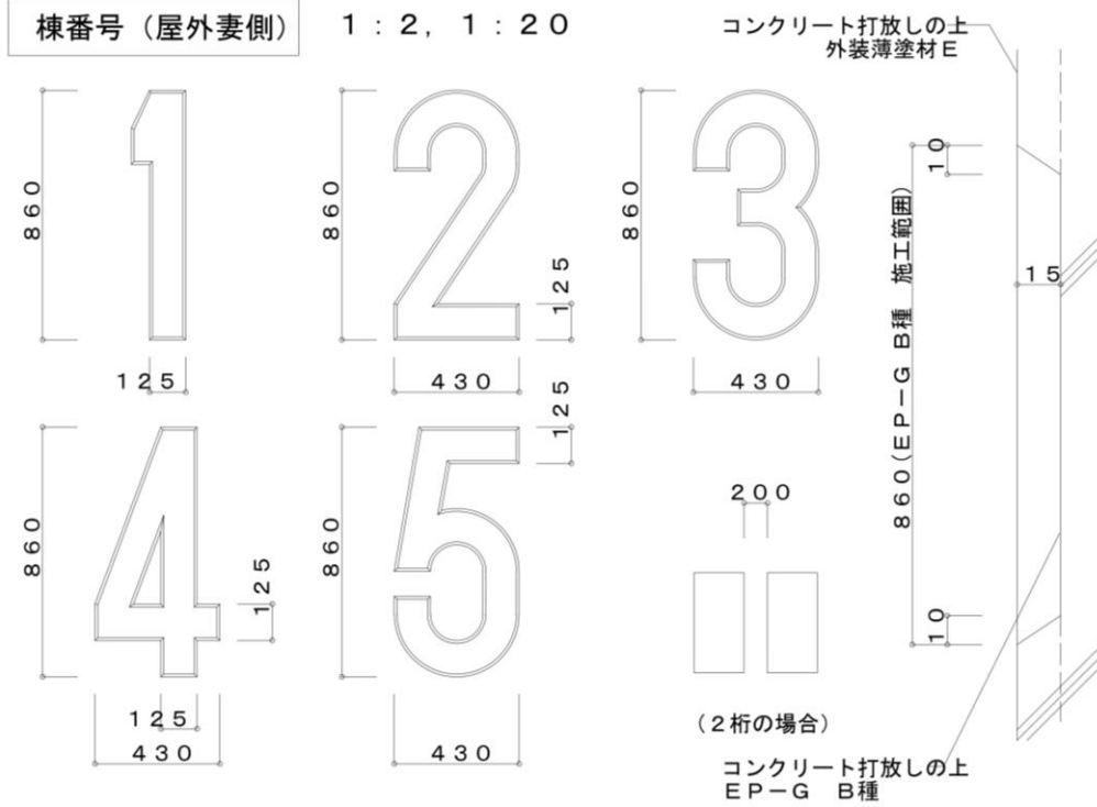
階数番号 (EVホール, 階段) 1 : 5
