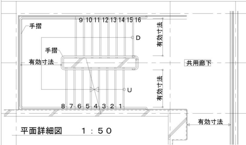
添付図 10 各部詳細図 (階段手摺 コンクリート手摺に取付る場合)
