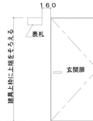
標準取付位置
