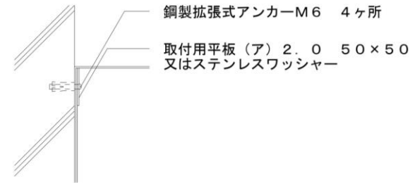
A 部 詳細図 1 : 5
