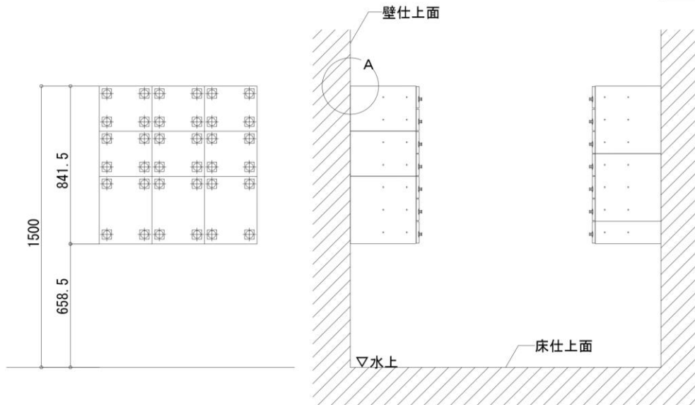
設置高さ位置図 1 : 20
