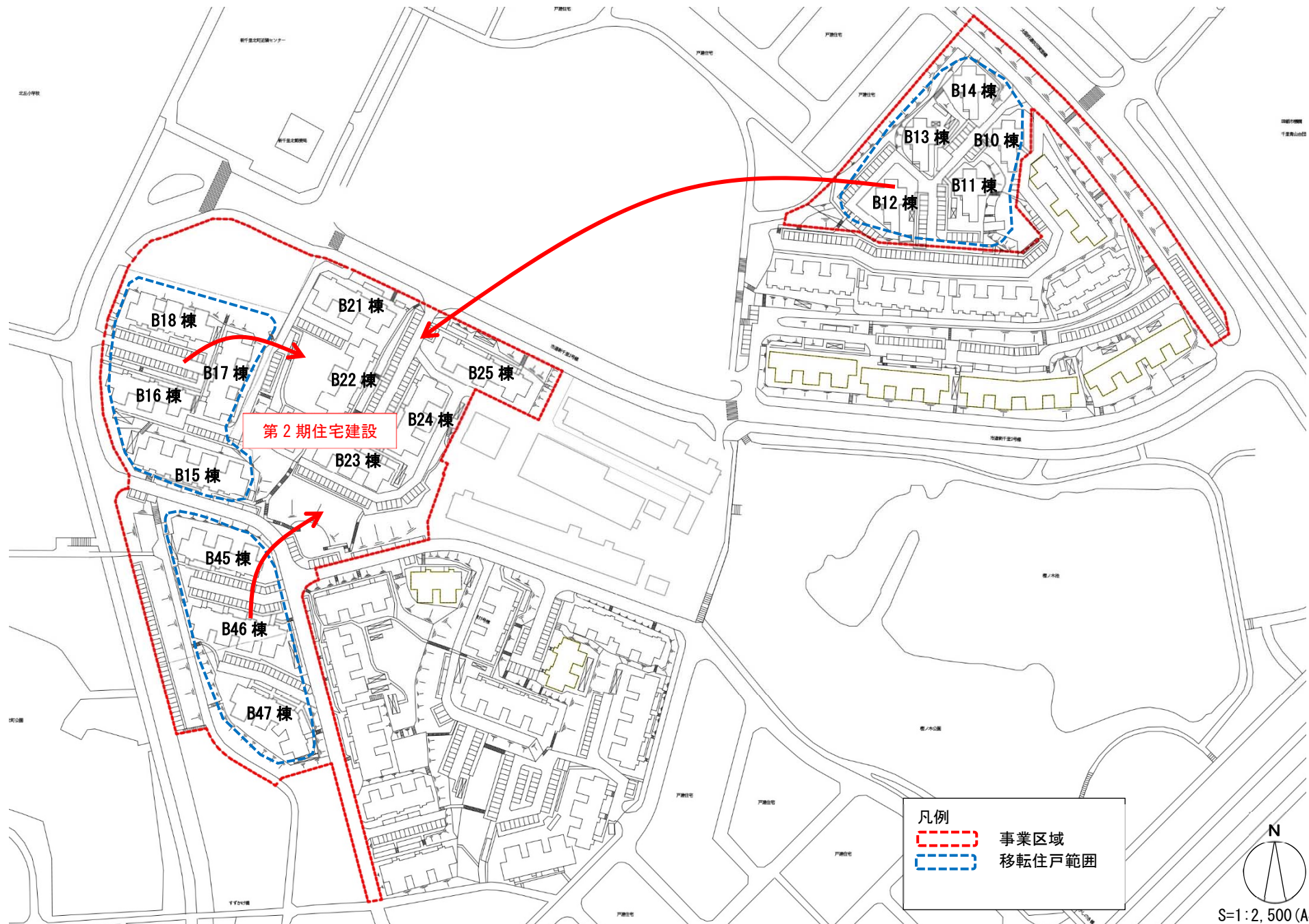
添付図2 大阪府営豊中新千里北第2期住宅 事業区域図・移転計画図
