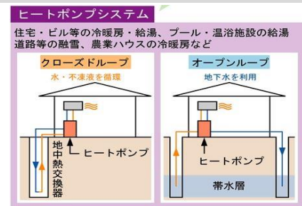
ヒートポンプシステムの図
