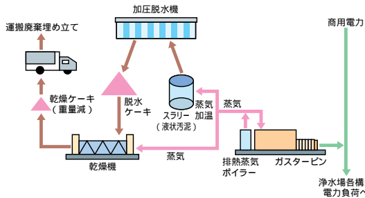
村野浄水場コージェネレーションシステムフロー
