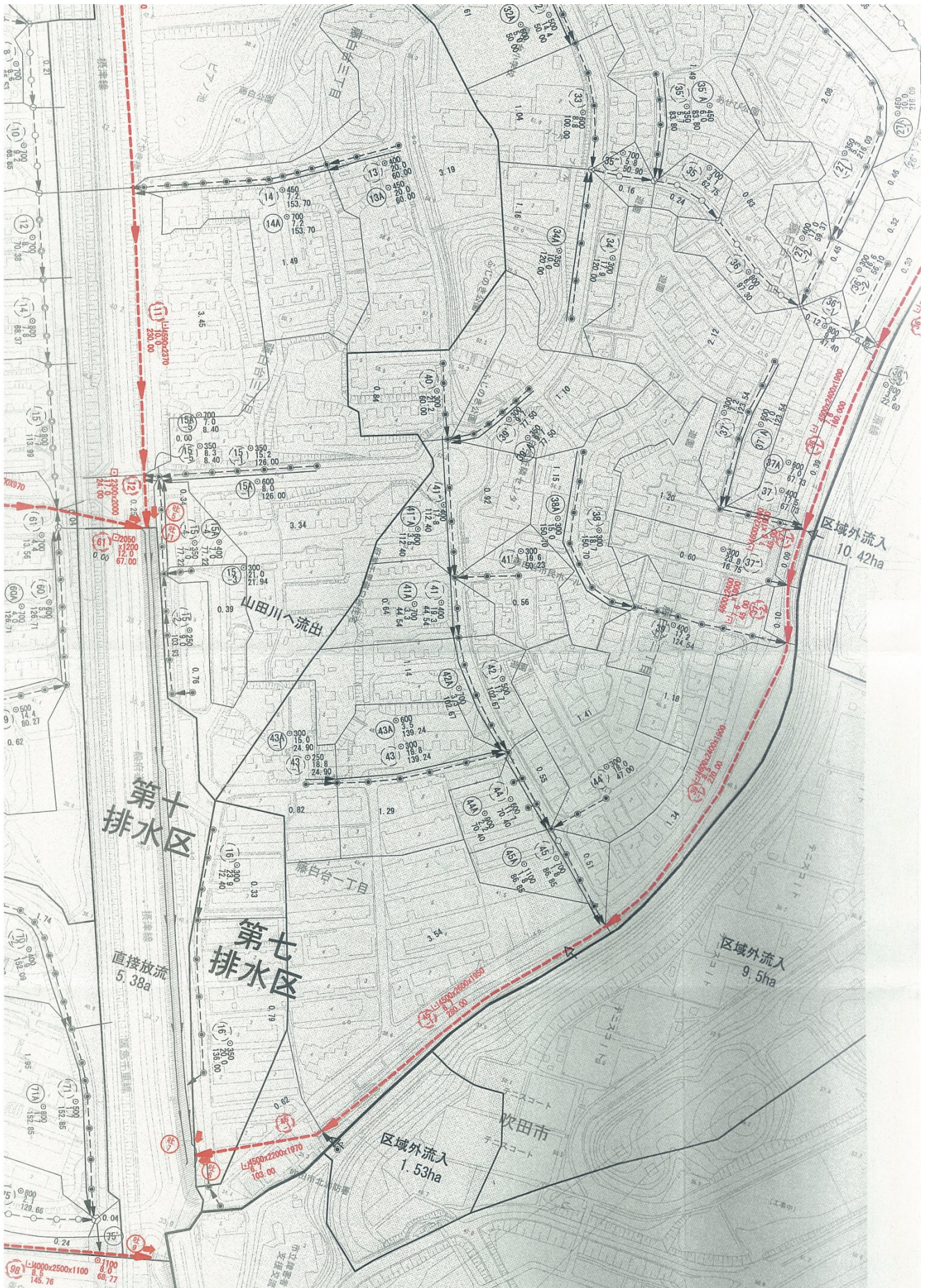
添付図14—吹田市下水道計画(雨水-部分)
