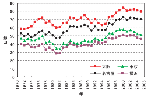
図-16 大都市における真夏日数 (5年移動平均)
