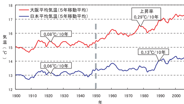
図-15 大阪・全国における年平均気温の推移 (5年移動平均)
