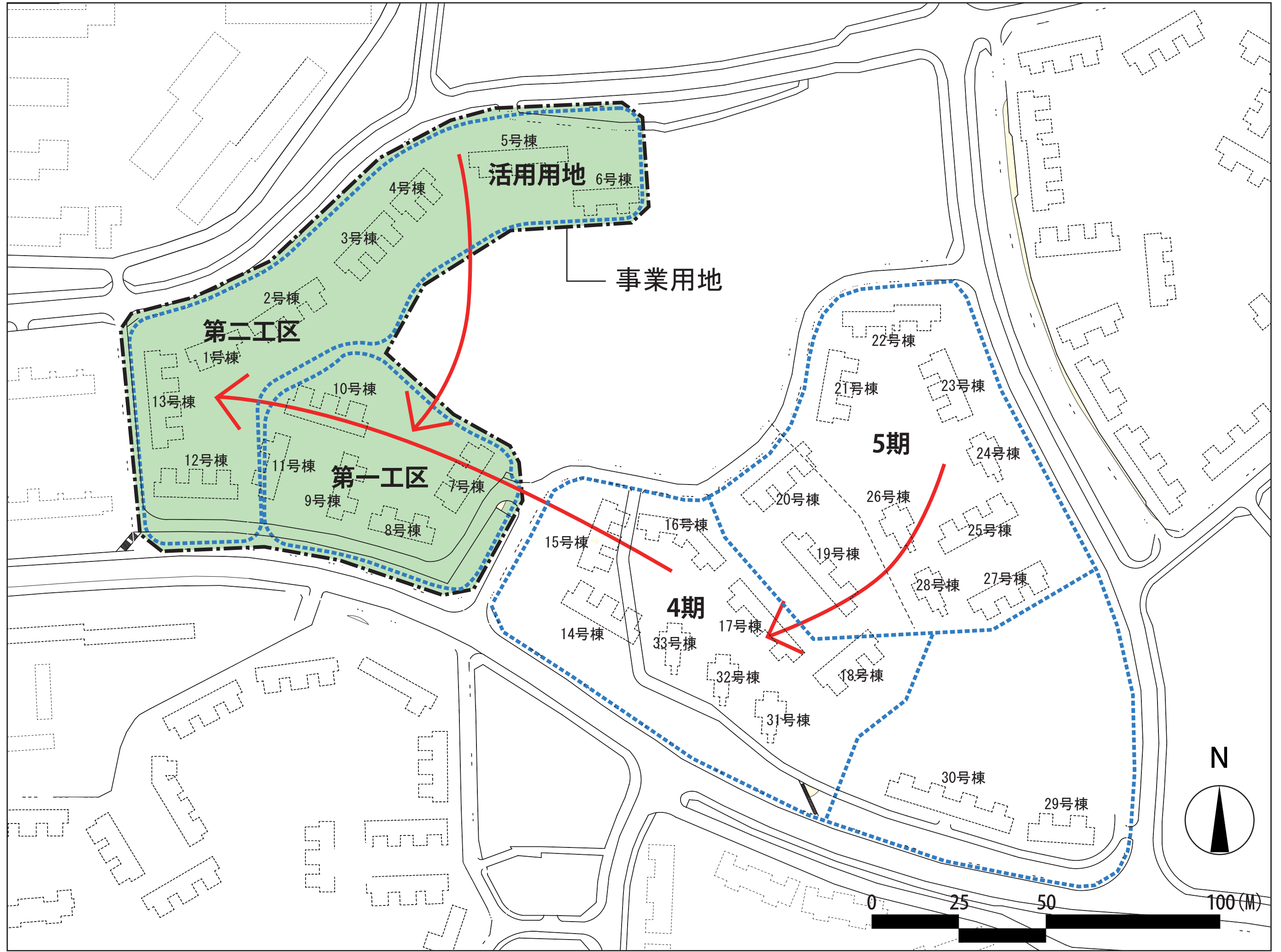
添付図2 移転計画図
