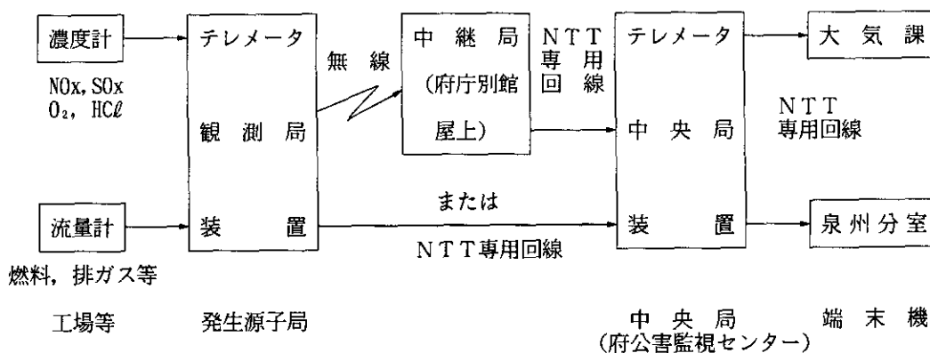
2-32図 大気汚染発生源常時監視システムの概要
